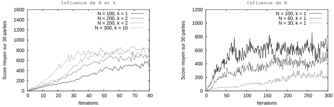
FIG. 3.4 – Gauche : 10 exécutions avec différentes valeurs de N et k sur 80 itérations, \rho = 0.1 et un bruit constant. Droite : 10 exécutions avec N \in \{30, 60, 100\} , k = 1 , \rho = 0.1 et un bruit constant sur 300 itérations.
