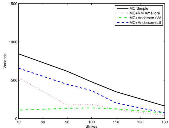
Erreurs relatives et variances des méthodes implémentées sur les options vanilles dans un marché très volatil ( \sigma = 0.3 ) d'actions à court terme
