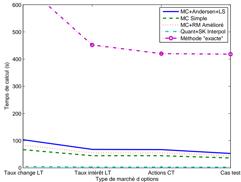
FIG. 3.2 – Temps de calcul des méthodes implémentées pour les options asiatiques
