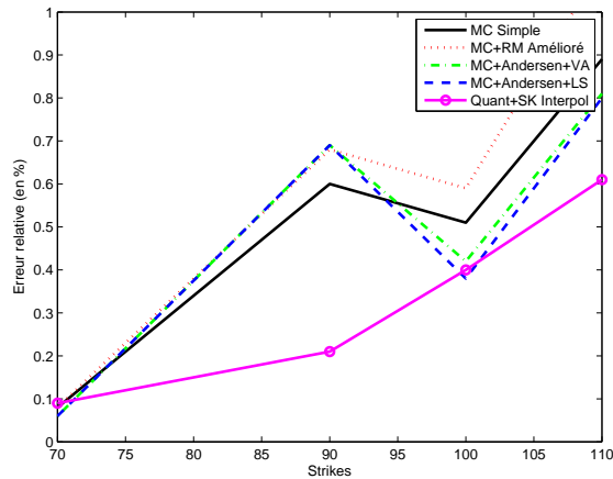
Erreurs relatives et variances des méthodes implémentées sur les options vanilles dans un cas test classique
