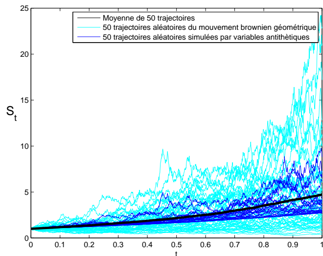
FIG. 1.3 – Effet de la technique des variables antithétiques sur les trajectoires simulées par Monte Carlo
