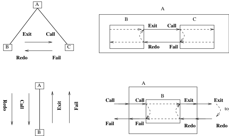
Fig. 7. Correspondance des représentations arbres /boîtes : combinaisons possibles des ports (boîtes adjacentes ou enchâssées)
