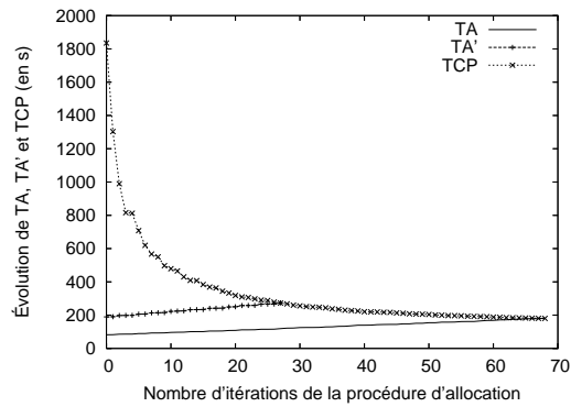
Figure 4. Exemple d'évolution de T_A , T'_A et de T_{CP} dans la procédure d'allocation de CPA et la nouvelle procédure d'allocation.
