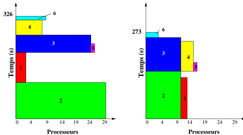
Figure 5. Ordonnancement du DAG de la figure 1 avec CPA (à gauche) et en utilisant la nouvelle allocation (à droite) sur une grappe homogène de 30 processeurs.
