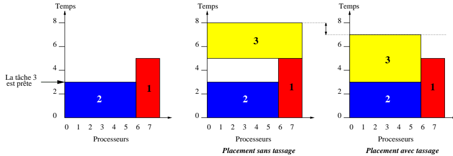
Figure 6. Illustration du placement avec tassage.
