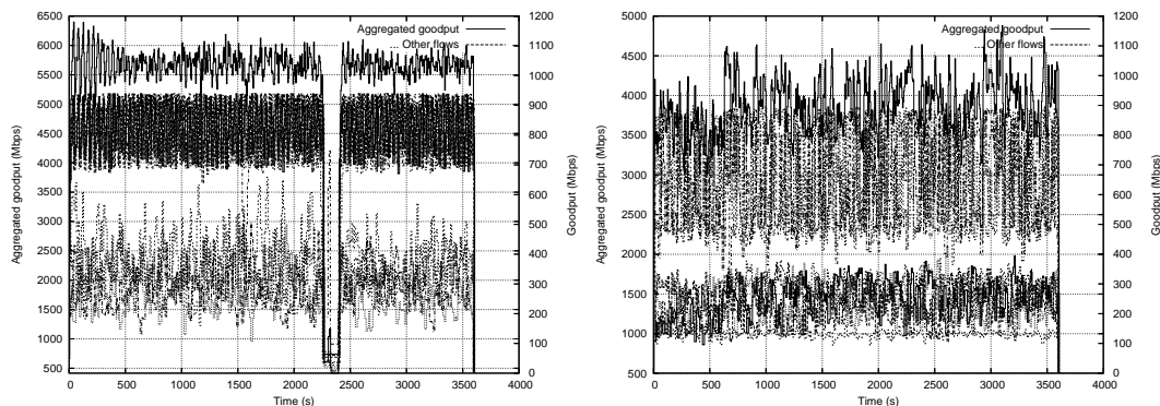
Figure 5: Bande passante agrègée obtenue de Sophia vers Rennes (et inversement) sur 10 flux.
