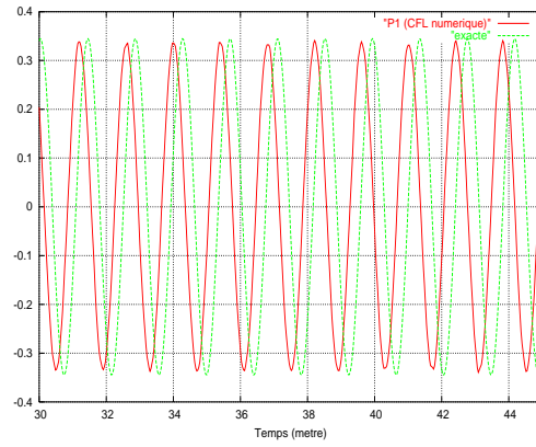
(b) Maillage 11 points par \lambda , CFL numérique
