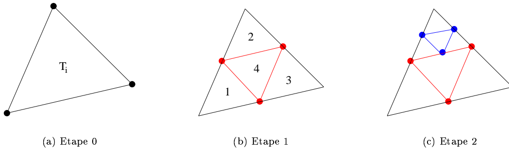
FIG. 3.3 – Les étapes de subdivision d’un triangle
