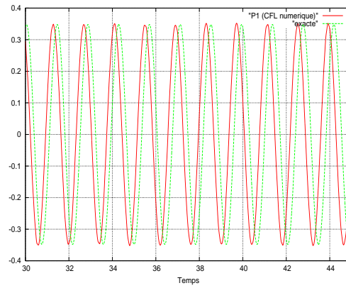
(b) Schéma GD- \mathbb{P}_1
