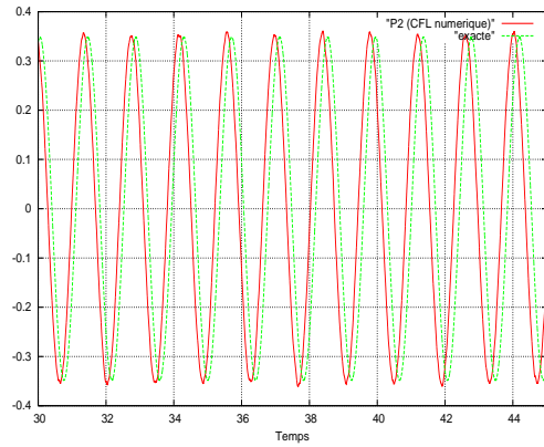
(c) Schéma GD- \mathbb{P}_2
