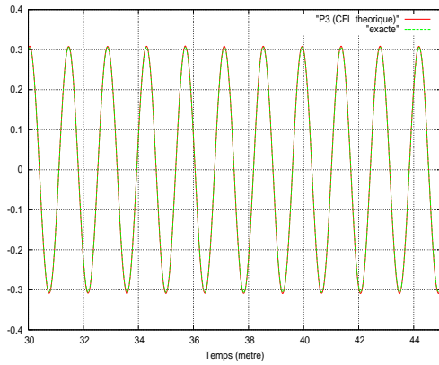
(a) Maillage 6 points par \lambda , CFL théorique
