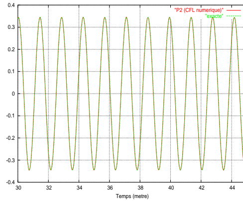
(d) Maillage 11 points par \lambda , CFL numérique
