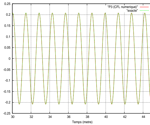
(d) Maillage 8 points par \lambda , CFL numérique
