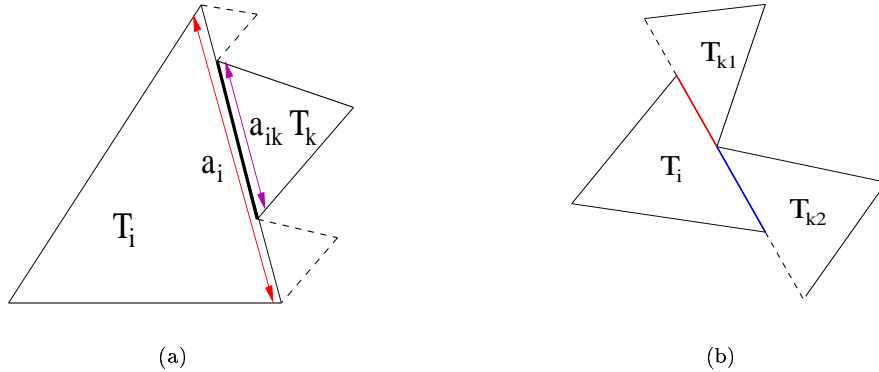
FIG. 3.2 – Deux types de non-conformité
