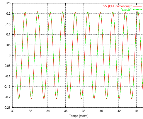
(b) Maillage 8 points par \lambda , CFL numérique
