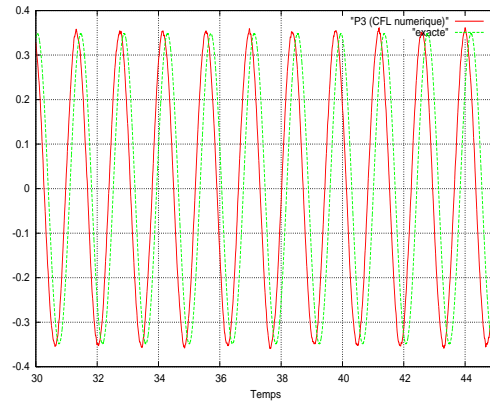
(d) Schéma GD- \mathbb{P}_3
