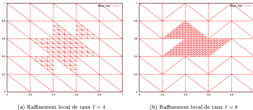
FIG. 3.4 – Exemples de raffinements locaux non-conforme d’un maillage triangulaire
