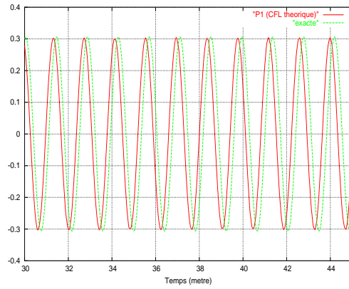
(c) Maillage 14 points par \lambda , CFL théorique
