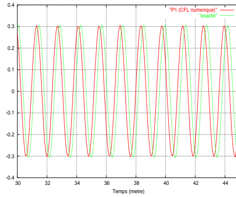
(d) Maillage 14 points par \lambda , CFL numérique
