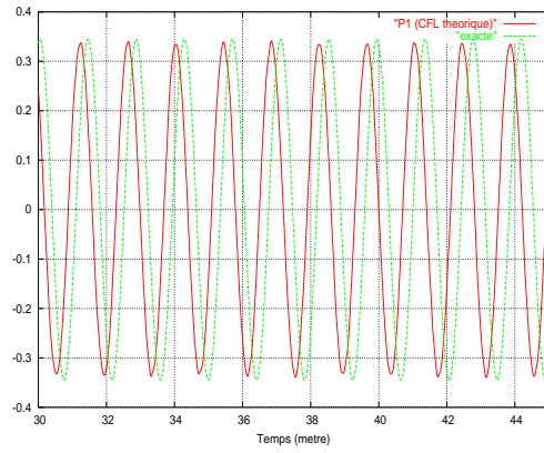
(a) Maillage 11 points par \lambda , CFL théorique
