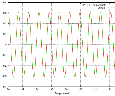
(b) Maillage 6 points par \lambda , CFL numérique
