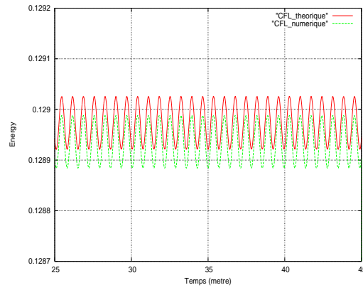
(d) GD- \mathbb{P}_3
