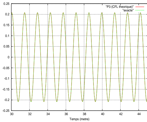
(c) Maillage 8 points par \lambda , CFL théorique
