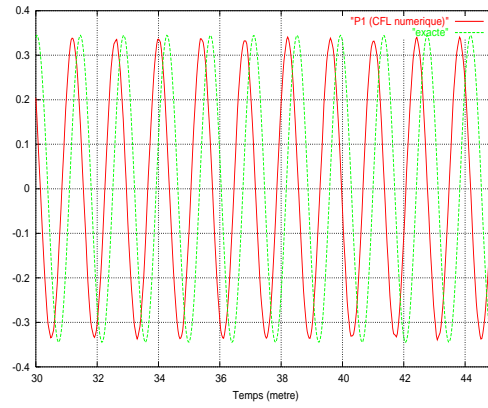
(b) Maillage 11 points par \lambda , CFL numérique
