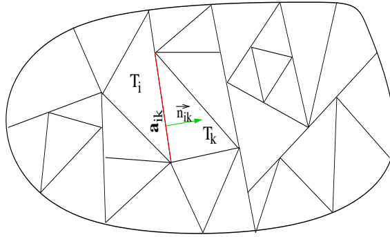
FIG. 2.1 – Maillage triangulaire non-conforme de \Omega
