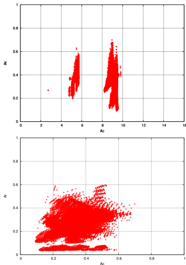
FIG. 1: Solutions inverses pour la voyelle [u] dans les plans X_c/A_c et A_c/A_l , où X_c est la position de la constriction principale mesurée comme la distance à la glotte le long du conduit, en cm, A_c l'aire à la constriction en cm^2 et A_l l'aire aux lèvres en cm^2 .
