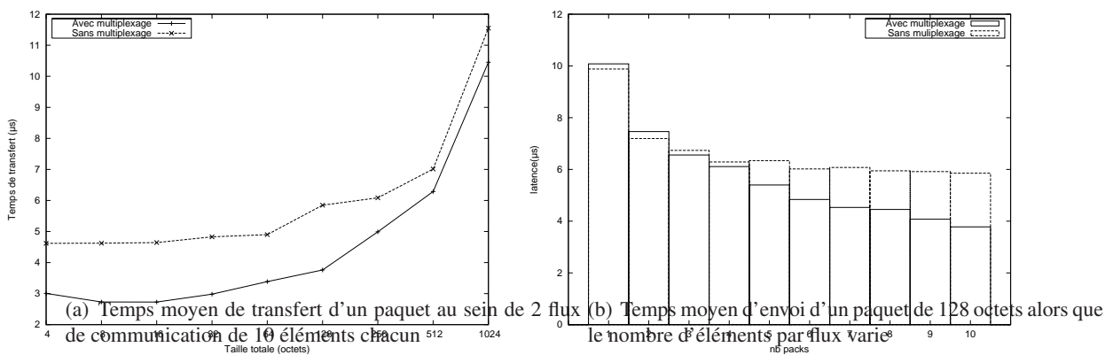
FIG. 6 – Multiplexage de 2 flux de n packs chacun. La masse effective transférée est de 2*n* taille considérée.
