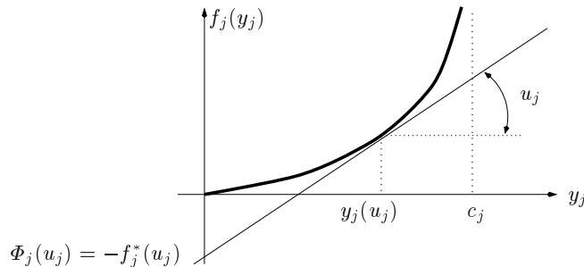
Fig. 2.1 Conjugating Kleinrock function
