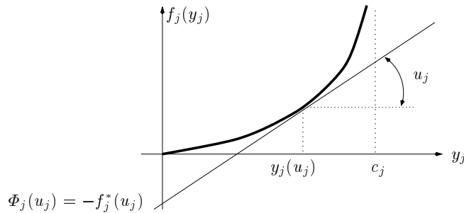
Fig. 2.1 Conjugating Kleinrock function
