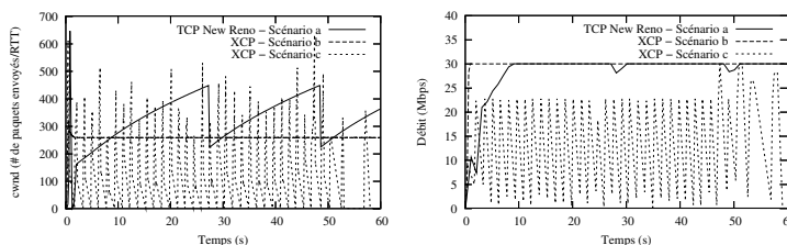
Figure 2. Évolution de la fenêtre de congestion et débit pour les scénarios a, b et c.
