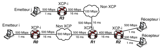
Figure 7. 2 files d'attente non-XCP partageant un chemin XCP
