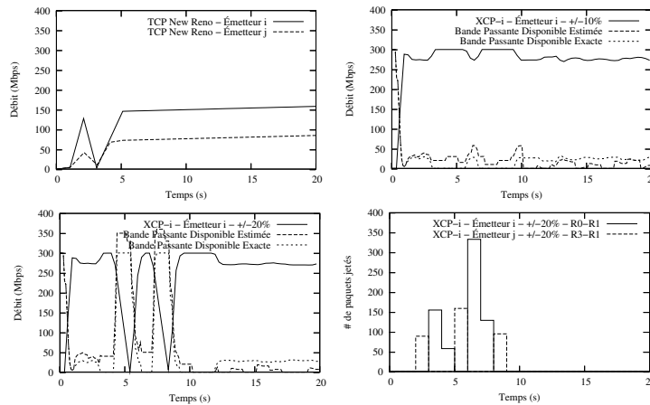
Figure 11. (h.g.) débit pour TCP. (h.d.) XCP-i, Emetteur i, 10%. (b.g) XCP-i, Emetteur i, 20%. (b.d.) pertes de paquets XCP-i, 20%
