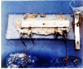
Le premier circuit intégré (Jack Kilby, 1958)
