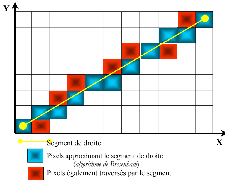
Figure 54 Discretisation d'un segment de droite.
