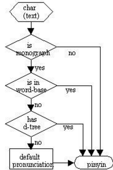
Figure 3.5 TTP conversion for Mandarin
