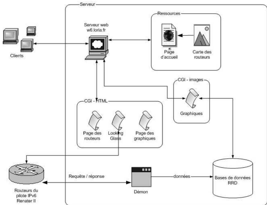
fig 7 : Architecture du site de supervision avant modification
