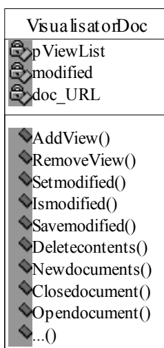
Fig. 19 : La classe VisualisatorDoc
