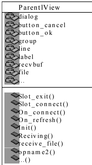
Fig. 20 : La classe ParentView
