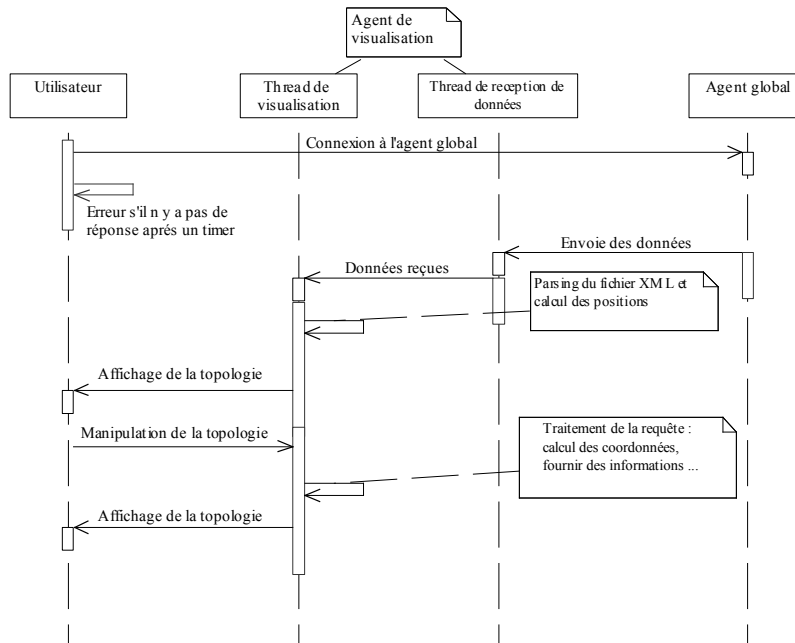
Fig. 14 : Fonctionnement du client : diagramme de séquences
