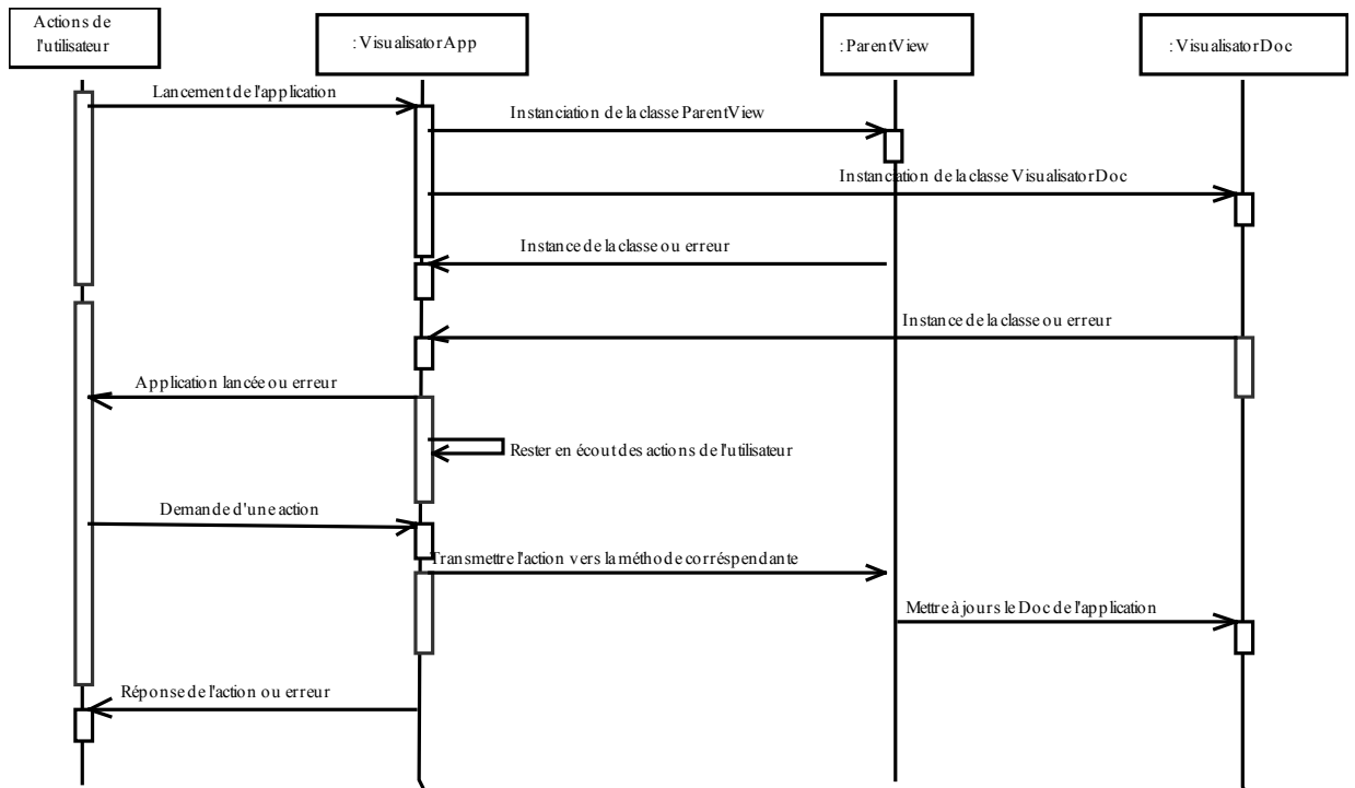
Fig. 21 : Diagramme des interactions entre classes
