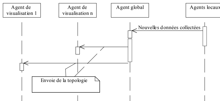
Fig. 12 : Gestion des rafraîchissements : diagramme de séquences
