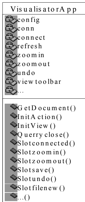
Fig. 18 : La classe VisualisatorApp
