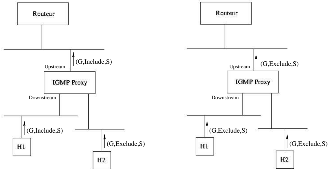
FIG. 5.3 – Filtrage sur les sources effectué pas le proxy IGMP
