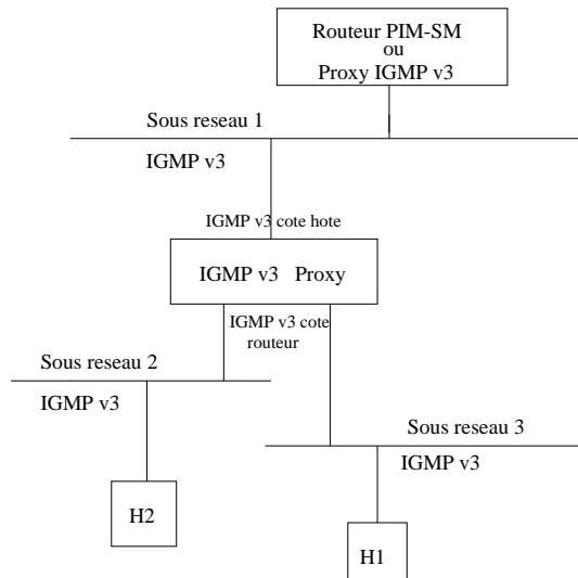
FIG. 5.1 – Architecture SSM utilisant un Proxy IGMPv3
