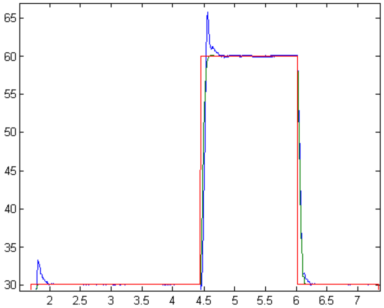
Fig. 7. Résultats en réponse à d'importants échelons d'amplitudes
