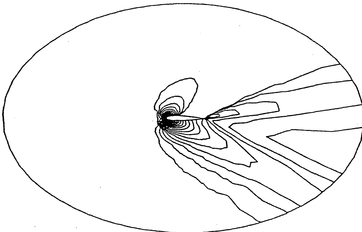
b) Isomach contours
