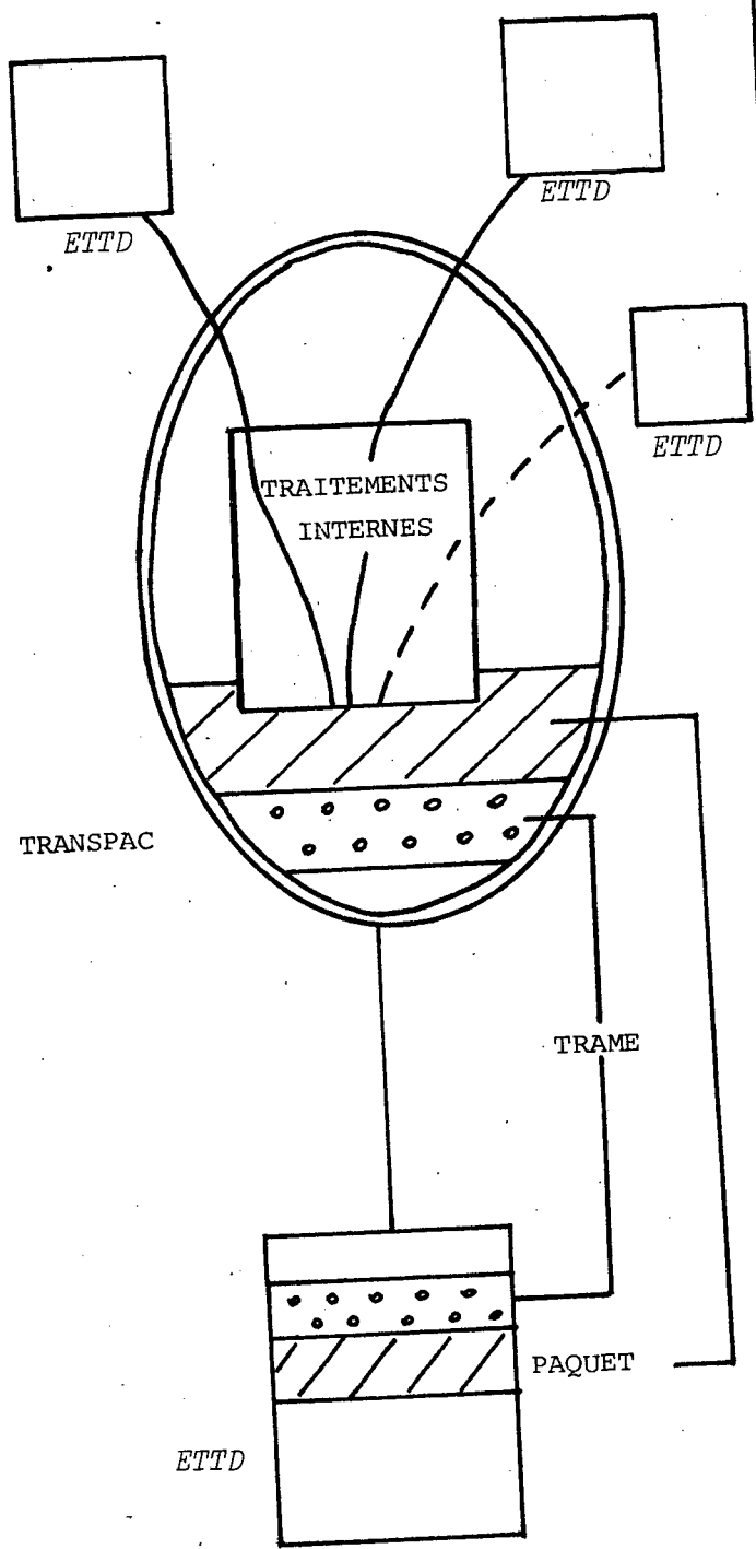
Figure II.5. - Différents niveaux des circuits virtuels.
