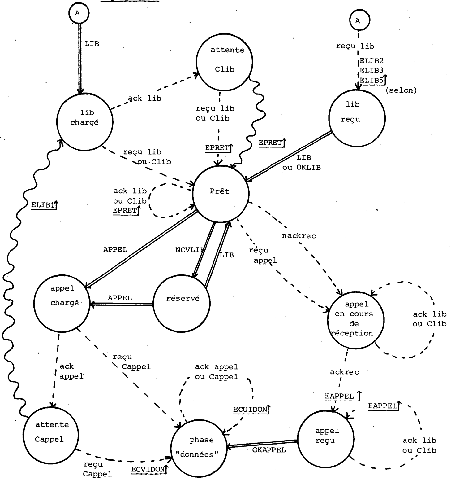
Figure IV.18. - AUTOMATE SIGNALISATION : ETABLISSEMENT ET LIBERATION.
