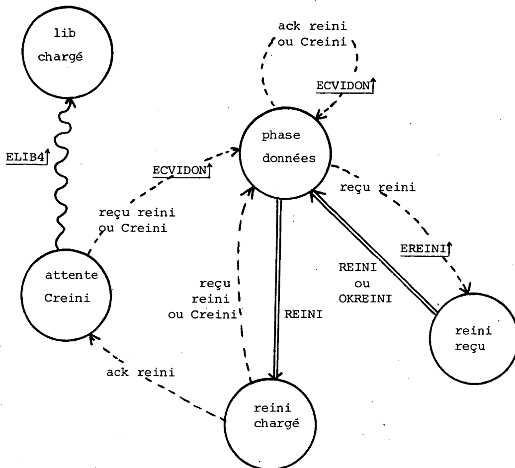
Figure IV.19. - AUTOMATE SIGNALISATION : REINITIALISATION.
