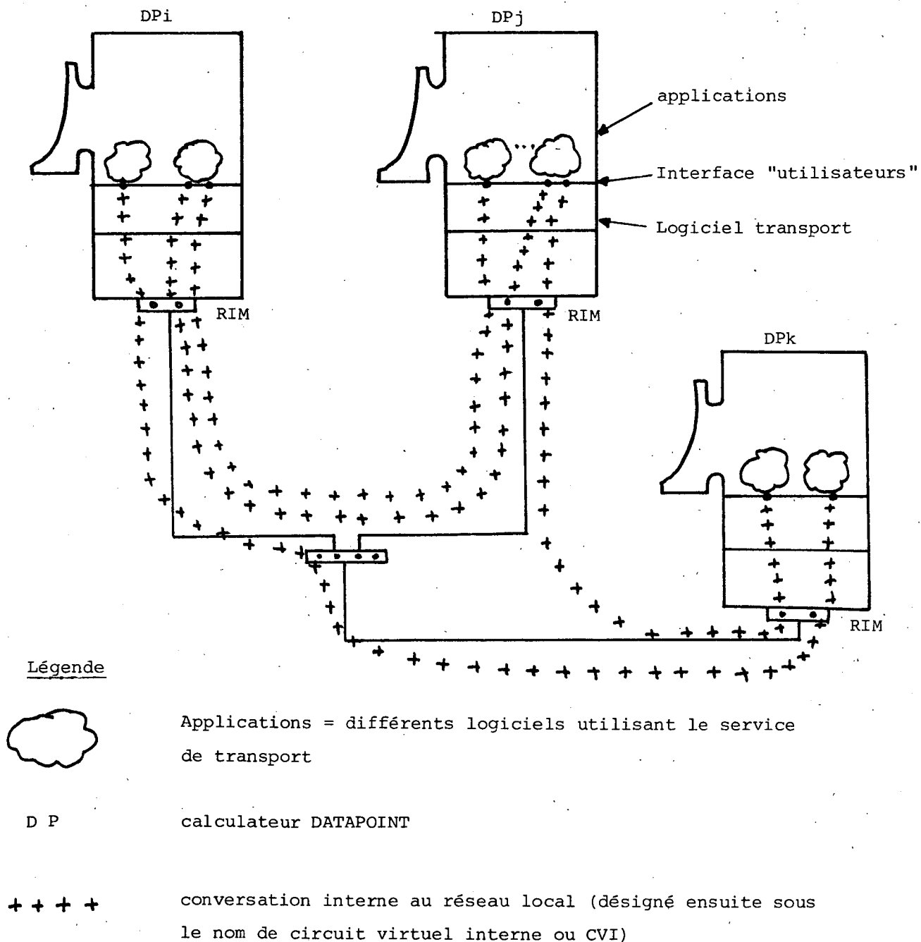
Figure I.1. - Conversations internes au réseau local.
