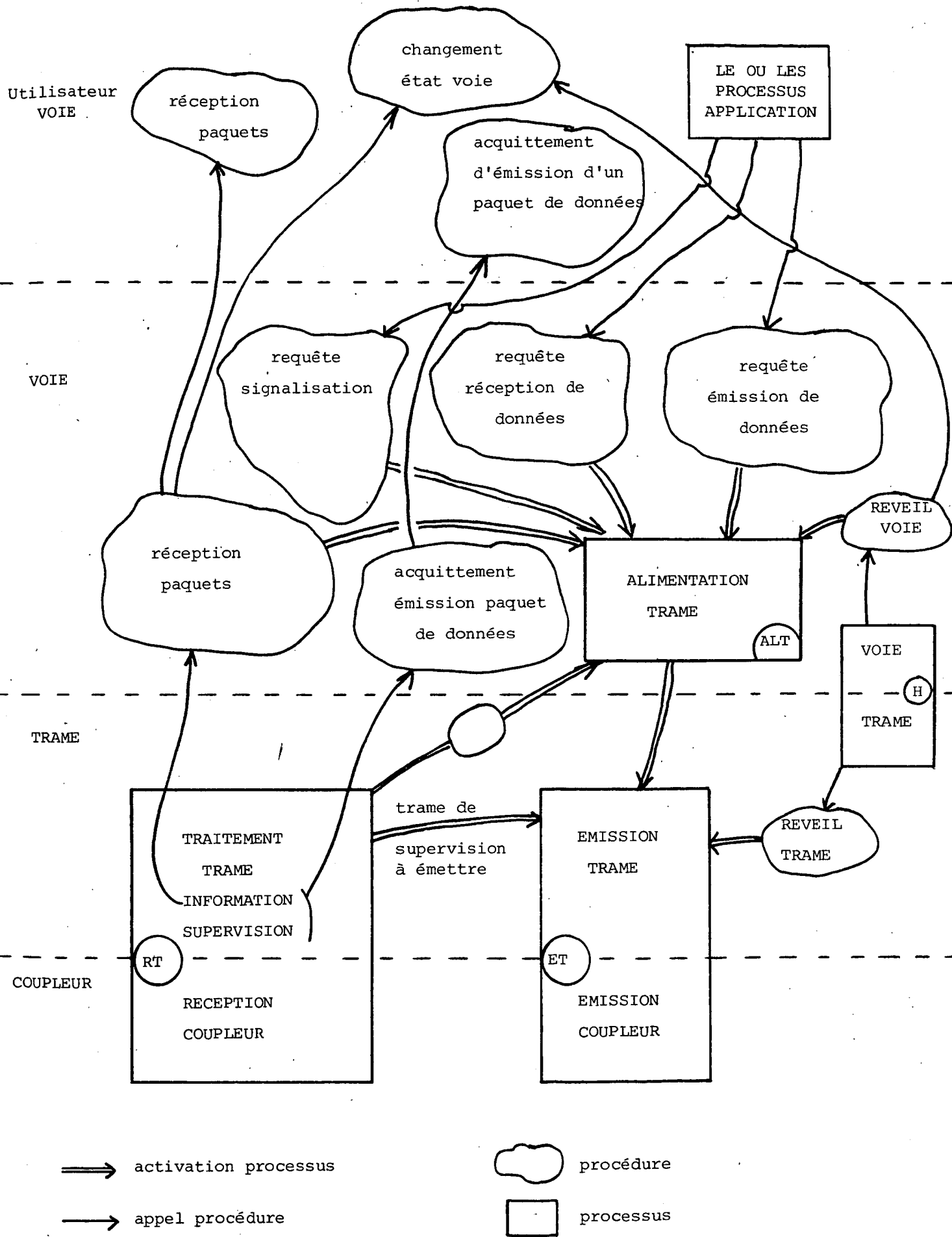
Figure III.11. - Logiciel CV
