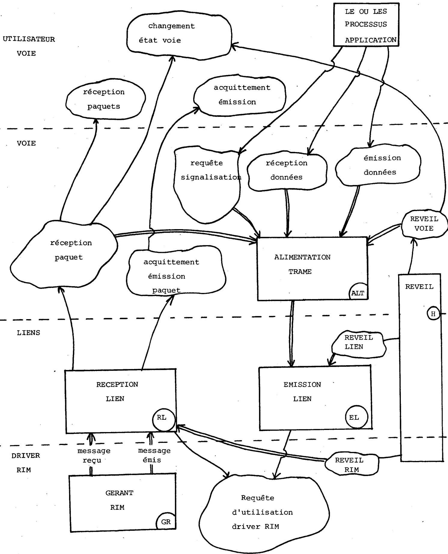
Figure III.12. - Logiciel CVI
