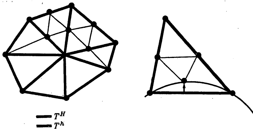
Figure 4 : subdivision
