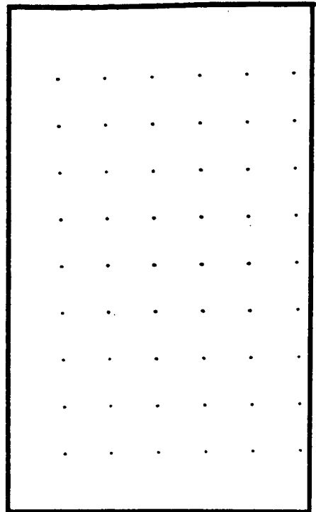
Fig. 8.c: Estimation error
