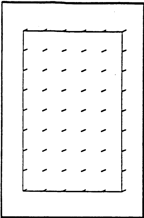
Fig. 8.a: True velocity
