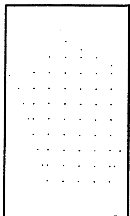
Fig. 10.f: Estimation error
