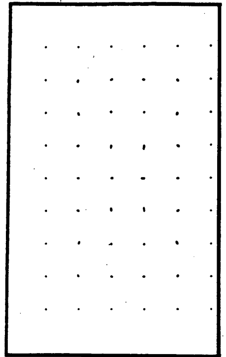
Fig. 11c: Estimation error
