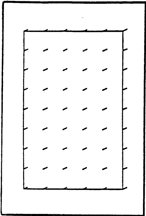
Fig. 7.a: True velocity
