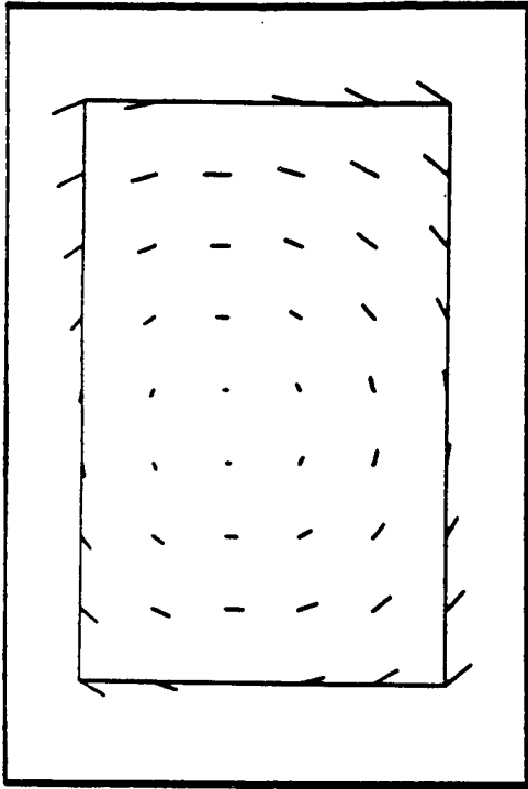
Fig. 12.a: True velocity
