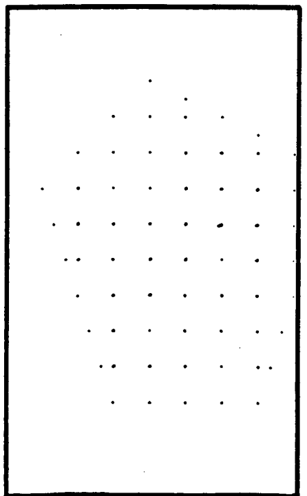
Fig. 8.f: Estimation error
