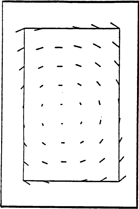
Fig. 9.a: True velocity
