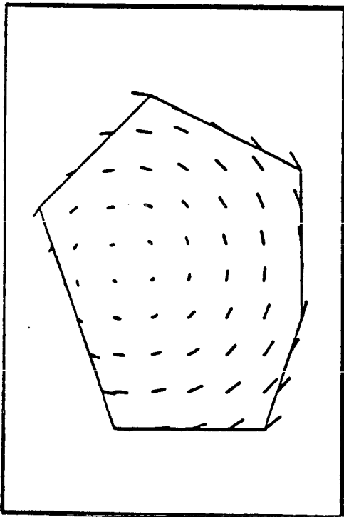
Fig. 9.d: True velocity
