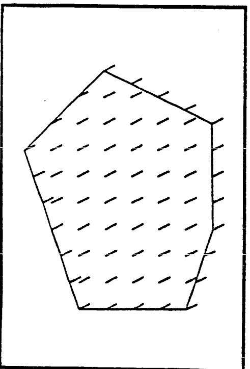
Fig. 7.d: True velocity
