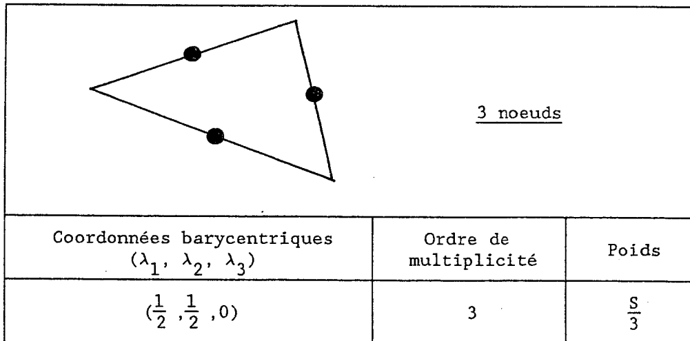
Figure 4.2.1 : Schéma d'intégration exact pour les polynômes de degré 2
