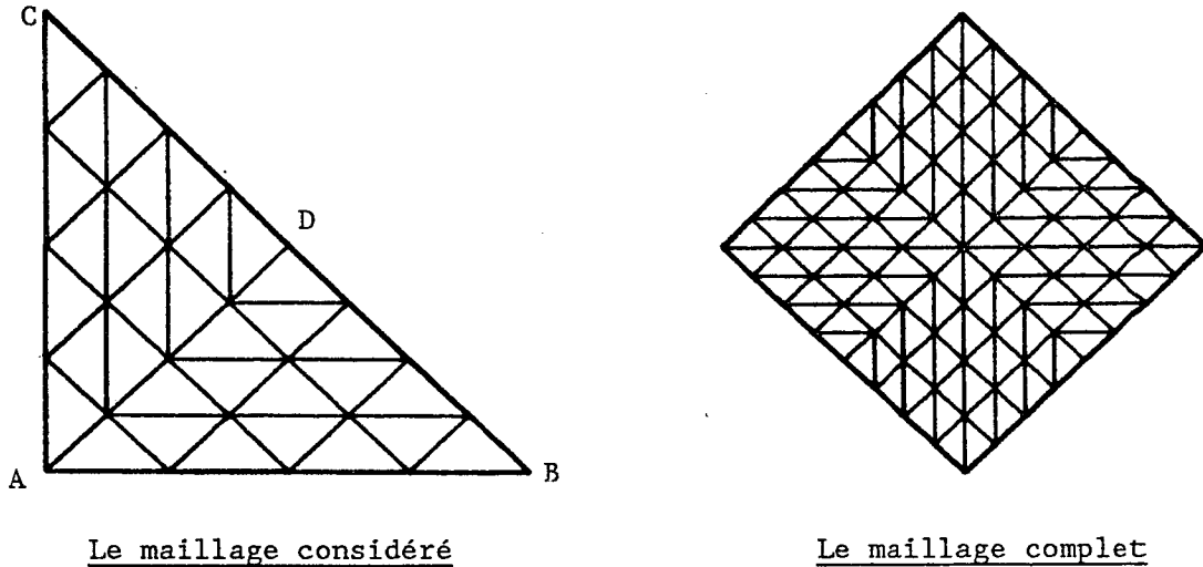
Figure 5.2.2 : les maillages
