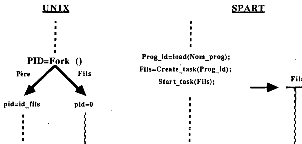
Figure 7: Comparaison de la création de processus.
