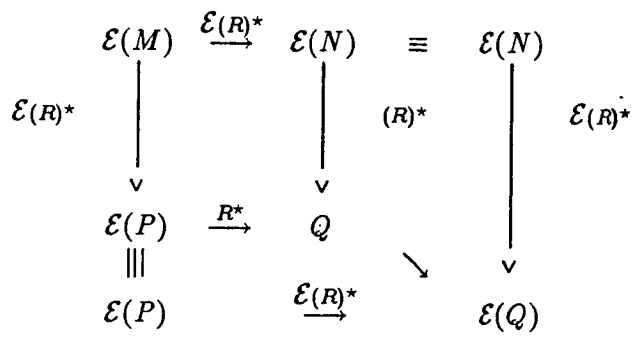
Figure 4: Confluence de \mathcal{E}(R)
