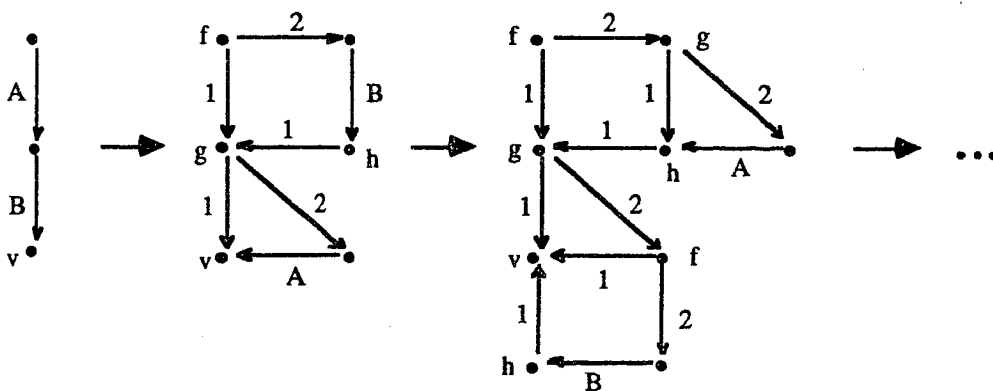
Fig. 3.2. Réécritures parallèles immédiates.
