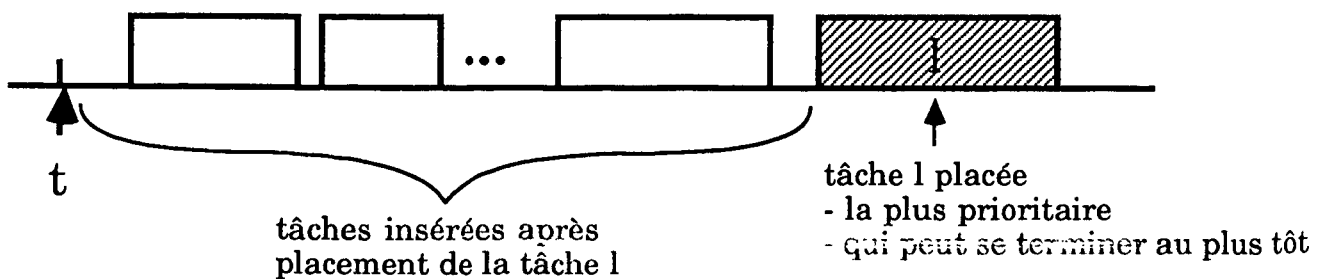
Fig. 1 Sous-ordonnement \Omega
