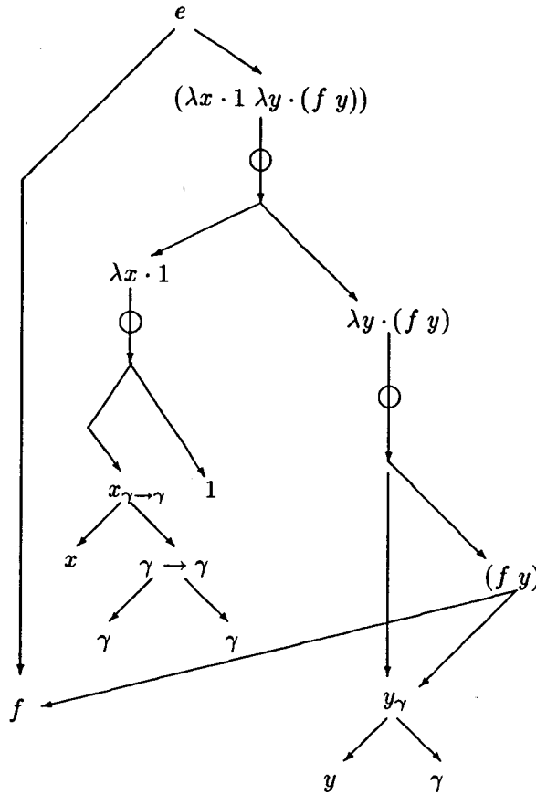
Figure 3 : Représentation interne de e := (f (\lambda x \cdot 1 f)) , f \in \mathcal{C} , \tau(f) = \gamma \rightarrow \gamma , x \in \mathcal{V}
