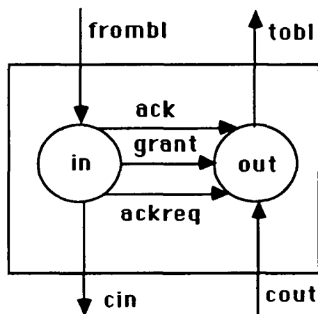
Fig. 16 Connecteur de bus physique
