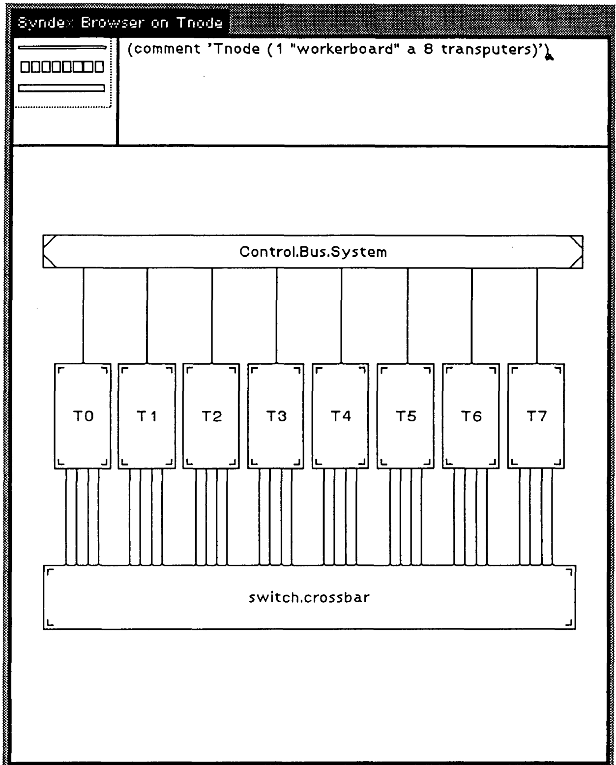
Fig. 25 SYNDEX Browser sur le TNODE
