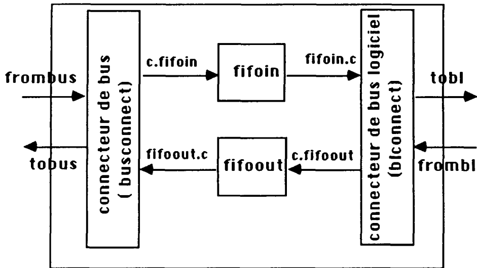
Fig. 15 Porte d'entrée - sortie
