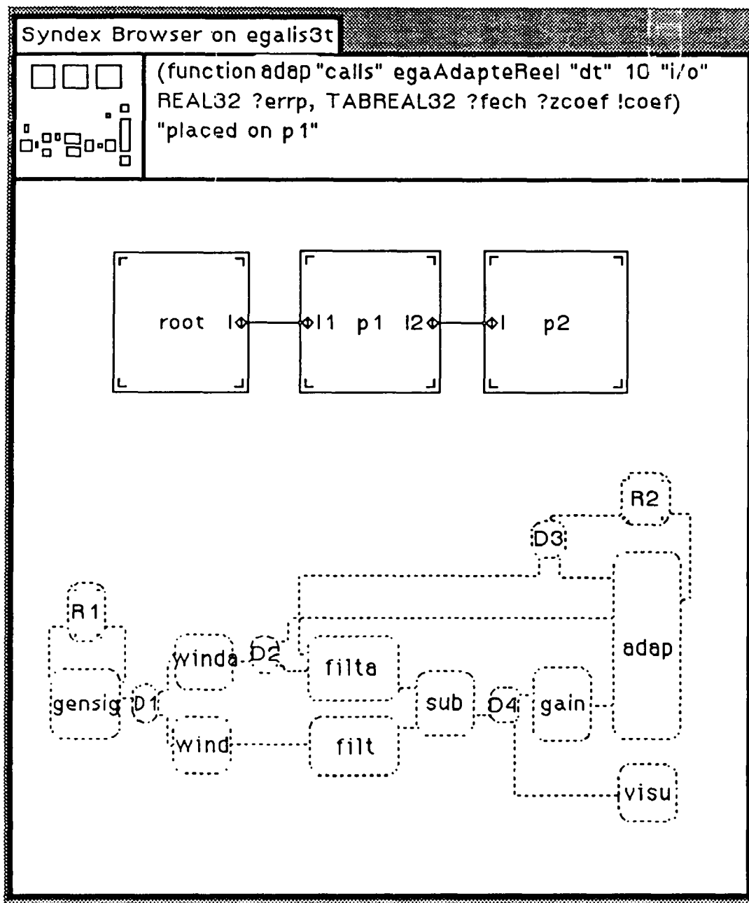
Fig. 22 SYNDEX Browser sur l'égaliseur adaptatif
