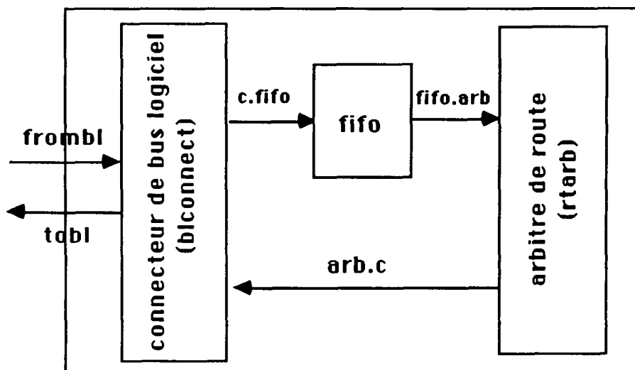
Fig. 14 Porte d'arbitrage de route
