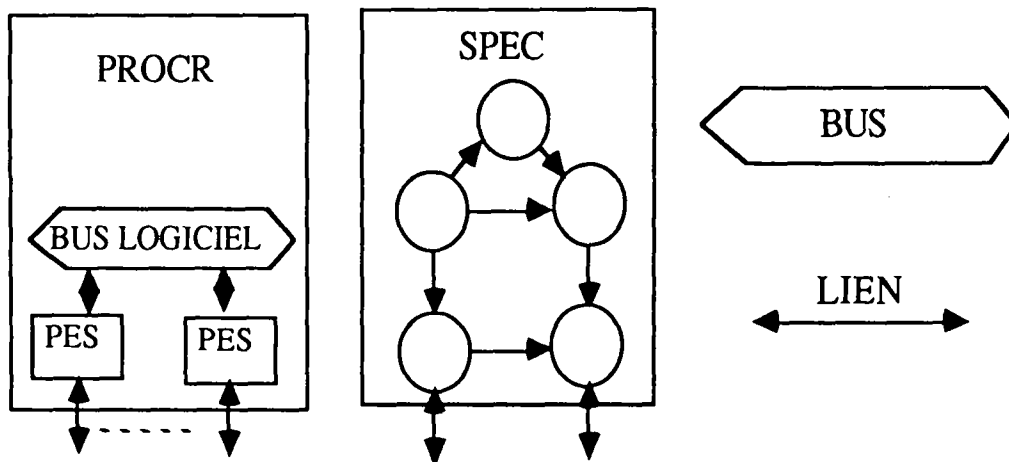
Fig. 5 Composant, bus et lien
