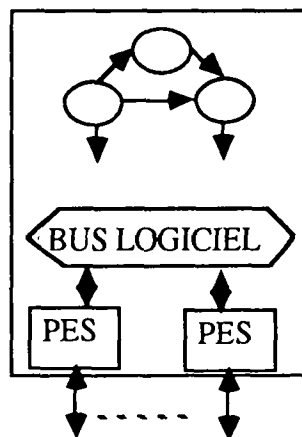
Fig. 8 Affectation d'un élément de partition à un processeur
