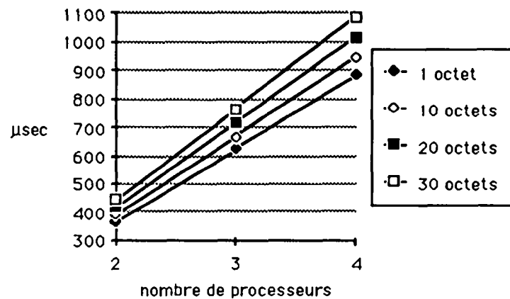
Fig. 21 Mesures sur une route en fonction du nombre de processeurs
