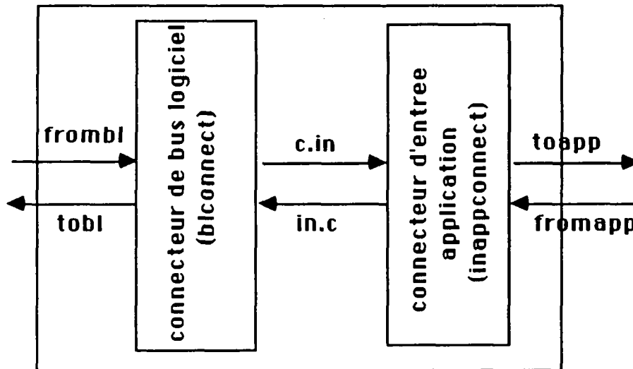
Fig. 13 Porte de réception
