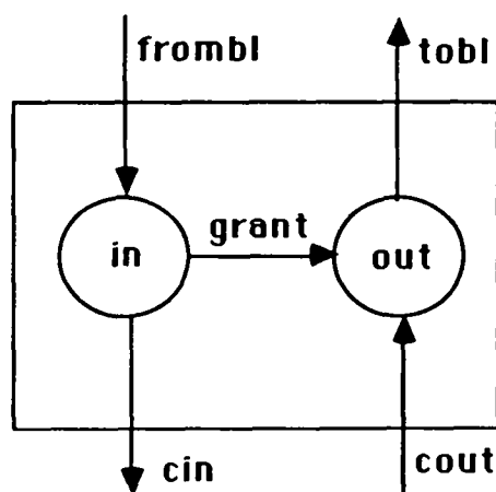
Fig. 12 Connecteur de bus logiciel
