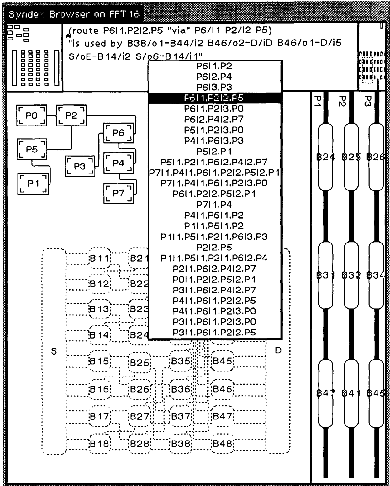
Fig. 24 SYNDEX Browser sur la FFT
