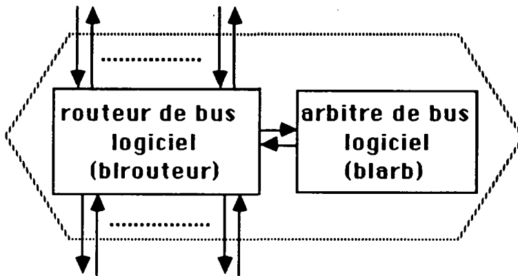
Fig. 18 Bus logiciel
