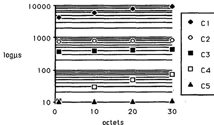
Fig. 19 Mesures entre deux transputers
