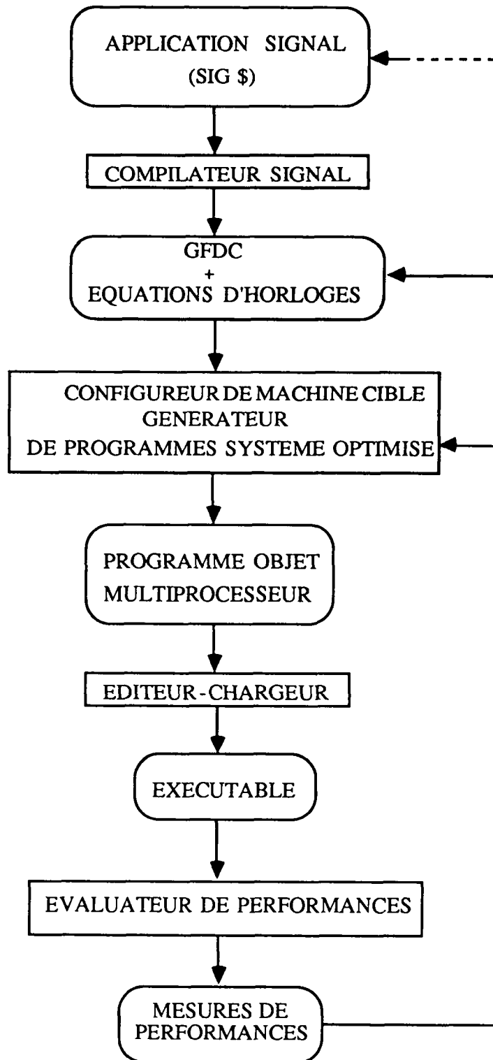
Fig. 1 Environnement SIGNAL SYNDEX
