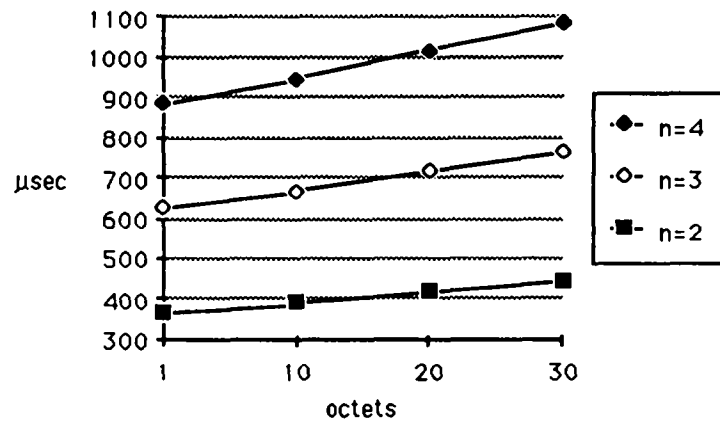
Fig. 20 Mesures sur une route en fonction de la longueur du message
