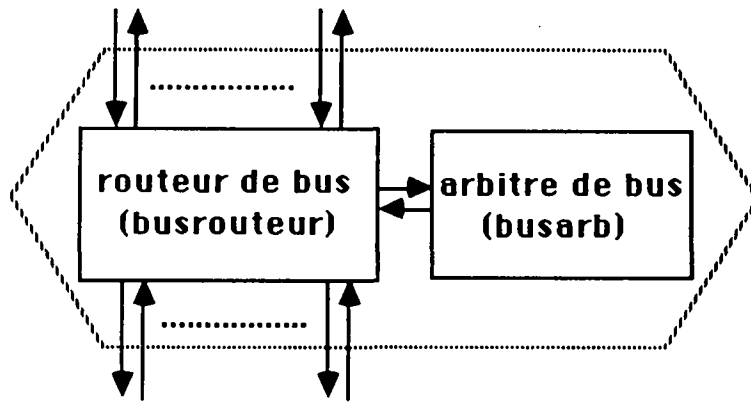
Fig. 17 Bus physique
