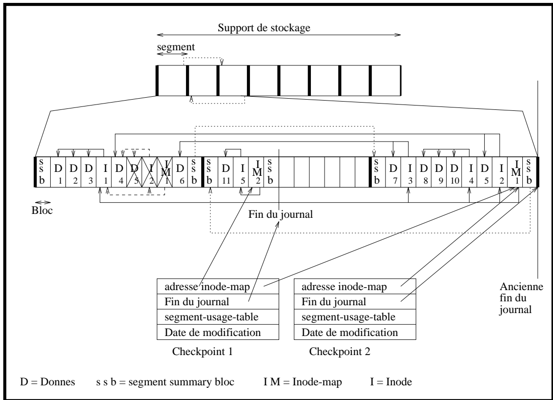
Figure III.2 : Structures d'inodes et d'inode-map dans LFS, système de fichier de Sprite
