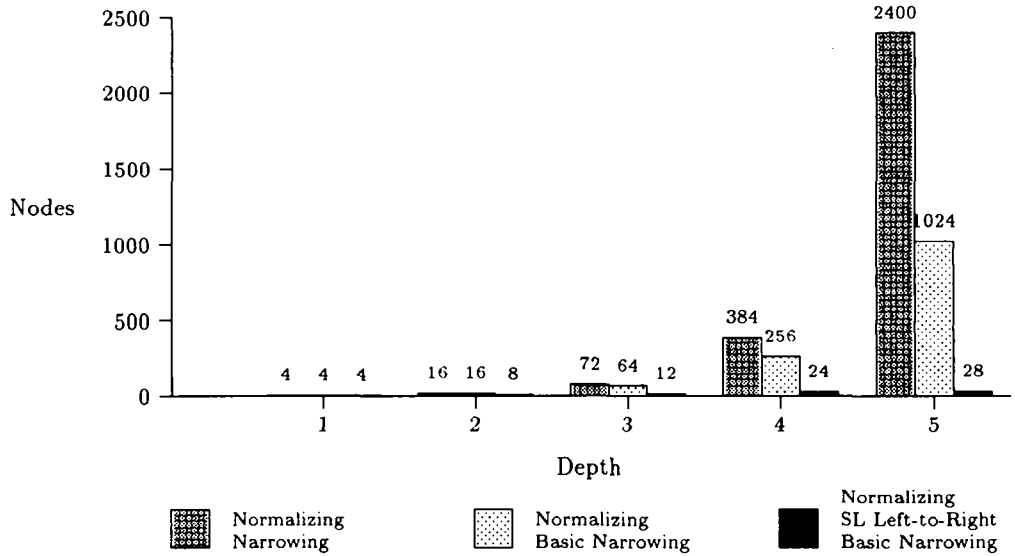
Fig. 4. Normalizing strategies
