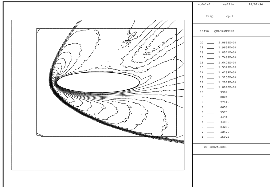
FIG. 17 - Lignes iso-Température
