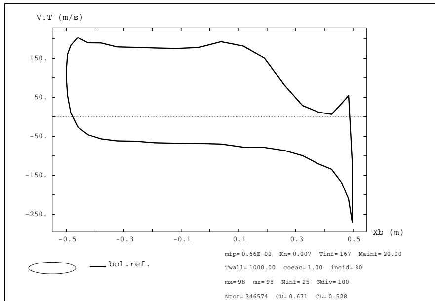
FIG. 13 - Vitesse tangentielle
