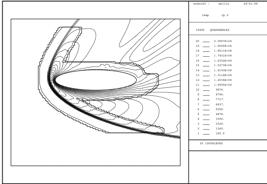
FIG. 29 - Lignes iso-Température
