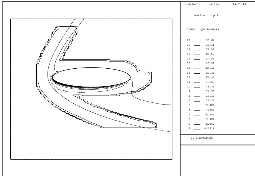
FIG. 30 - Lignes iso-densité
