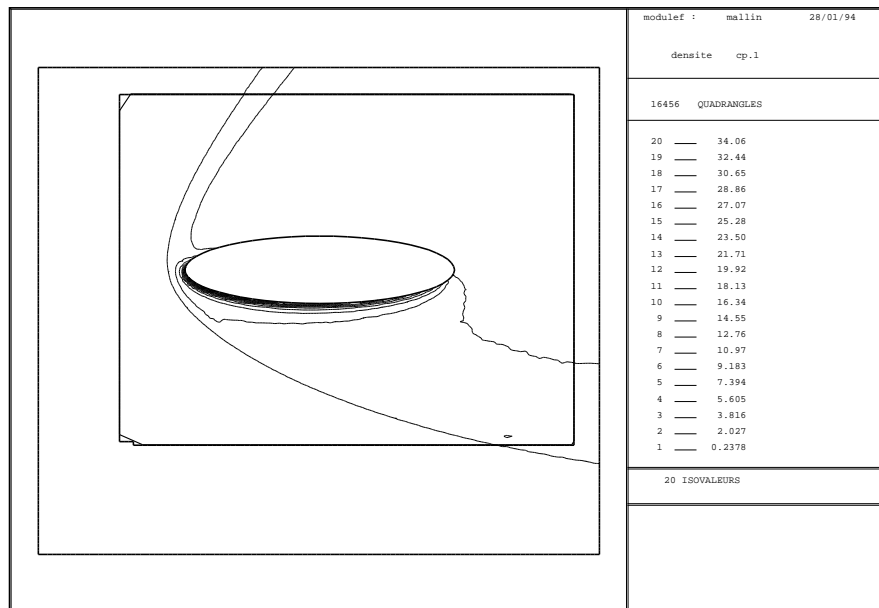
FIG. 18 - Lignes iso-densité
