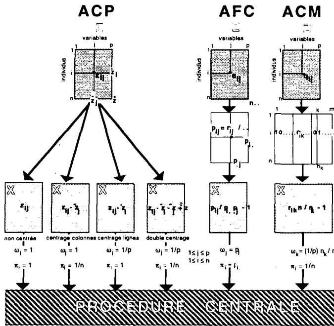
Figure-7 Codage, transformation des données initiales et matrices de pondération, [DOLE91].
