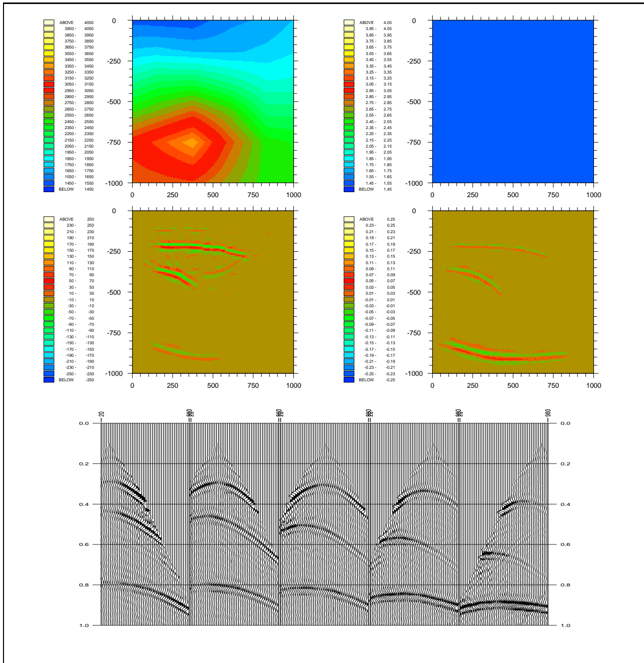
FIG. 24 – Resimulation des données après minimisation par rapport à l'échelle 1 du propagateur à partir du propagateur optimal à l'échelle 0. Pour les sections en temps, axe horizontal: position des récepteurs (m), axe vertical: temps (s). Pour les sections en profondeur, axe horizontal: distance horizontale (m), axe vertical: altitude (m). La vitesse est en m/s et l'impédance en 10^6 \text{ kg/m}^2\text{s} . Haut: propagateur optimal à l'échelle 1 (gauche), impédance lisse constante 1,5. Milieu: estimation intermédiaire de la réflectivité en profondeur relative à la vitesse r_v (gauche) et à l'impédance r_\sigma (droite). Bas: resimulation dans le milieu (\pi_1^* + r_v, 1.5 + r_\sigma) .
