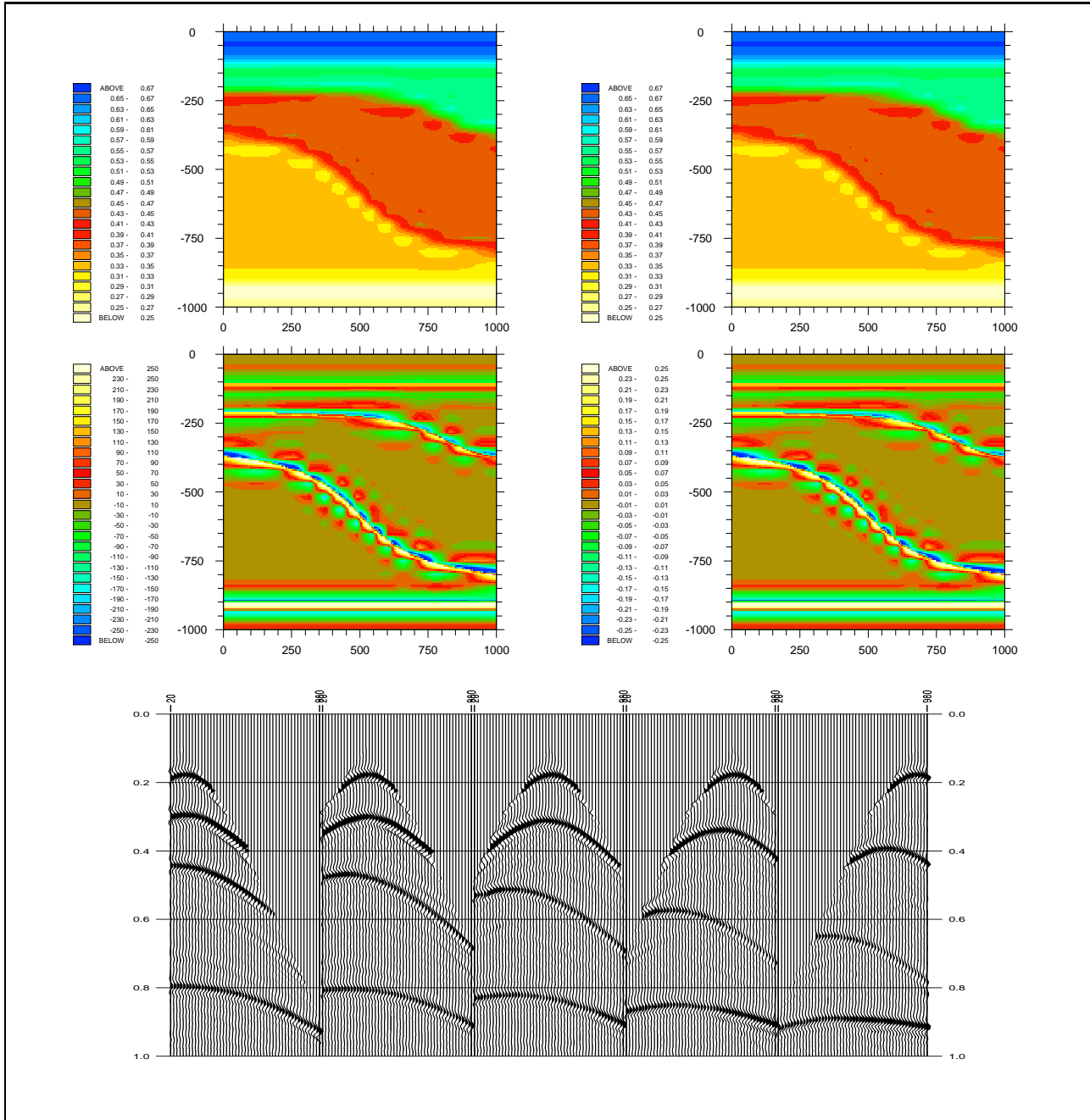
FIG. 16 – Simulation dans le “vrai” milieu. Pour les sections en temps, axe horizontal : position des récepteurs, axe vertical : temps (s). Pour les sections en profondeur, axe horizontal : distance horizontale (m), axe vertical : altitude (m). Les lenteurs sont en 10^{-3} s/m et les impédances en 10^6 kg/m 2 s. Haut : “vraie” lenteur lisse \bar{v}_s (gauche) et “vraie” impédance lisse \bar{\sigma}_s (droite). Milieu : “vraie” lenteur rugueuse \bar{v}_r (gauche) et “vraie” impédance rugueuse \bar{\sigma}_r (droite). Bas : simulation dans le milieu ( \bar{v}_s + \bar{v}_r, \bar{\sigma}_s + \bar{\sigma}_r ).
