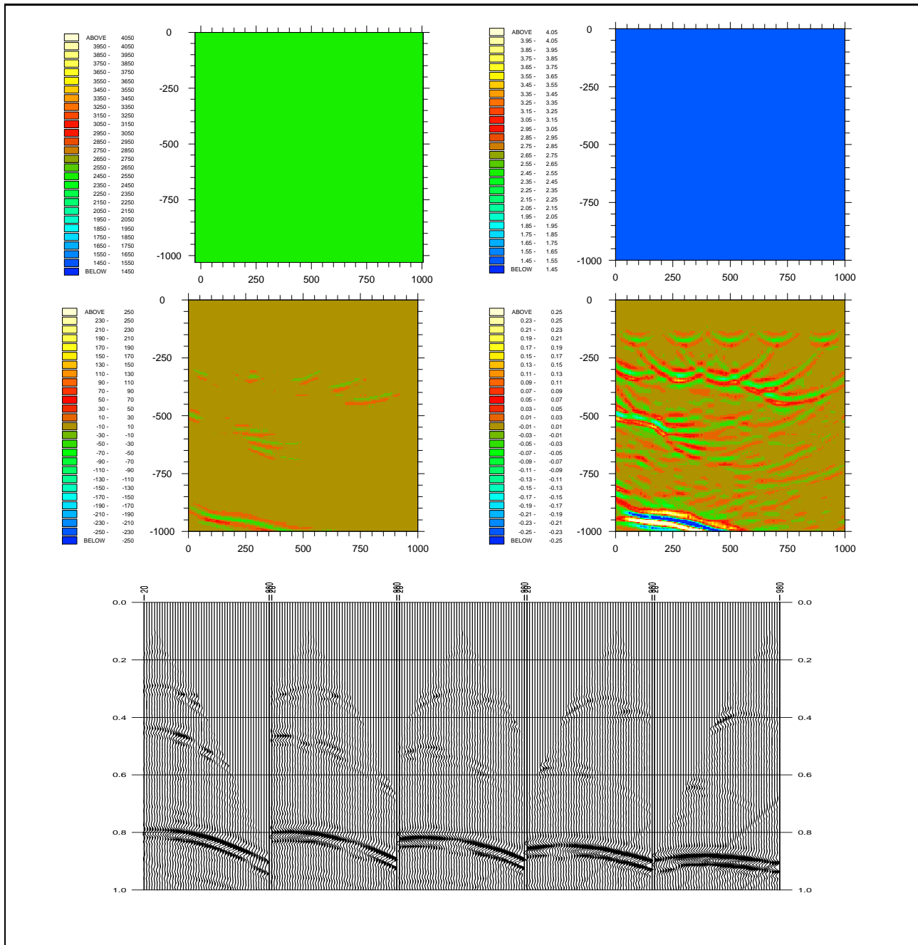
FIG. 22 – Resimulation des données avec le propagateur initial. Pour les sections en temps, axe horizontal : position des récepteurs (m), axe vertical : temps (s). Pour les sections en profondeur, axe horizontal : distance horizontale (m), axe vertical : altitude (m). La vitesse est en m/s et l'impédance en 10^6 \text{ kg/m}^2 \text{ s} . Haut : propagateur initial 2500 (gauche), impédance lisse constante 1,5. Milieu : estimation intermédiaire de la réflectivité en profondeur relative à la vitesse r_v (gauche) et à l'impédance r_\sigma (droite). Bas : resimulation dans le milieu (2500 + r_v, 1.5 + r_\sigma) .
