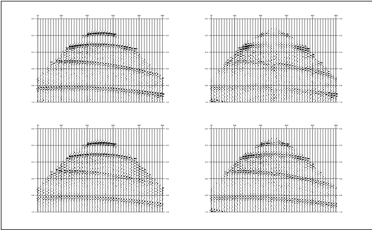
FIG. 21 – Estimation de la “vraie” réflectivité en temps par minimisation par rapport à s avec le “vrai” propagateur. Axe horizontal : position des récepteurs (m), axe vertical : temps (s). Haut : réflectivité en temps initiale s^0 = d = \varphi(\bar{v}, \bar{\sigma}) (gauche), resimulation initiale \mathcal{M}\varphi(\bar{\pi}, s^0) . Bas : réflectivité en temps après 24 itérations de minimisation s^{24} (gauche), resimulation correspondante \mathcal{M}\varphi(\bar{\pi}, s^{24}) .
