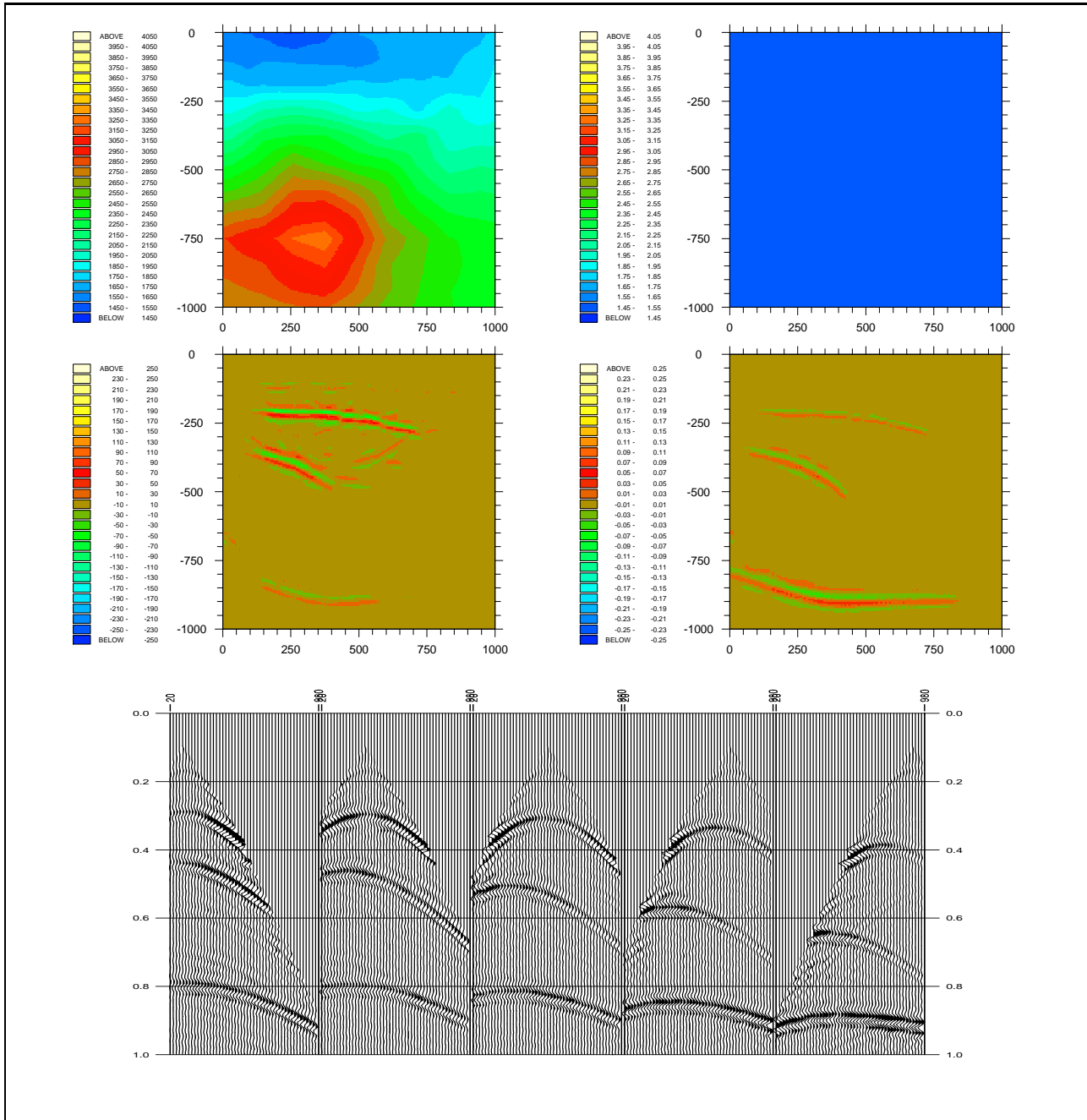
FIG. 26 – Resimulation des données après minimisation par rapport à l'échelle 3 du propagateur à partir du propagateur optimal à l'échelle 2. Pour les sections en temps, axe horizontal: position des récepteurs (m), axe vertical: temps (s). Pour les sections en profondeur, axe horizontal: distance horizontale (m), axe vertical: altitude (m). La vitesse est en m/s et l'impédance en 10^6 \text{ kg/m}^2\text{s} . Haut: propagateur optimal à l'échelle 3 (gauche), impédance lisse constante 1,5. Milieu: estimation intermédiaire de la réflectivité en profondeur relative à la vitesse r_v (gauche) et à l'impédance r_\sigma (droite). Bas: resimulation dans le milieu (\pi_3^* + r_v, 1.5 + r_\sigma) .
