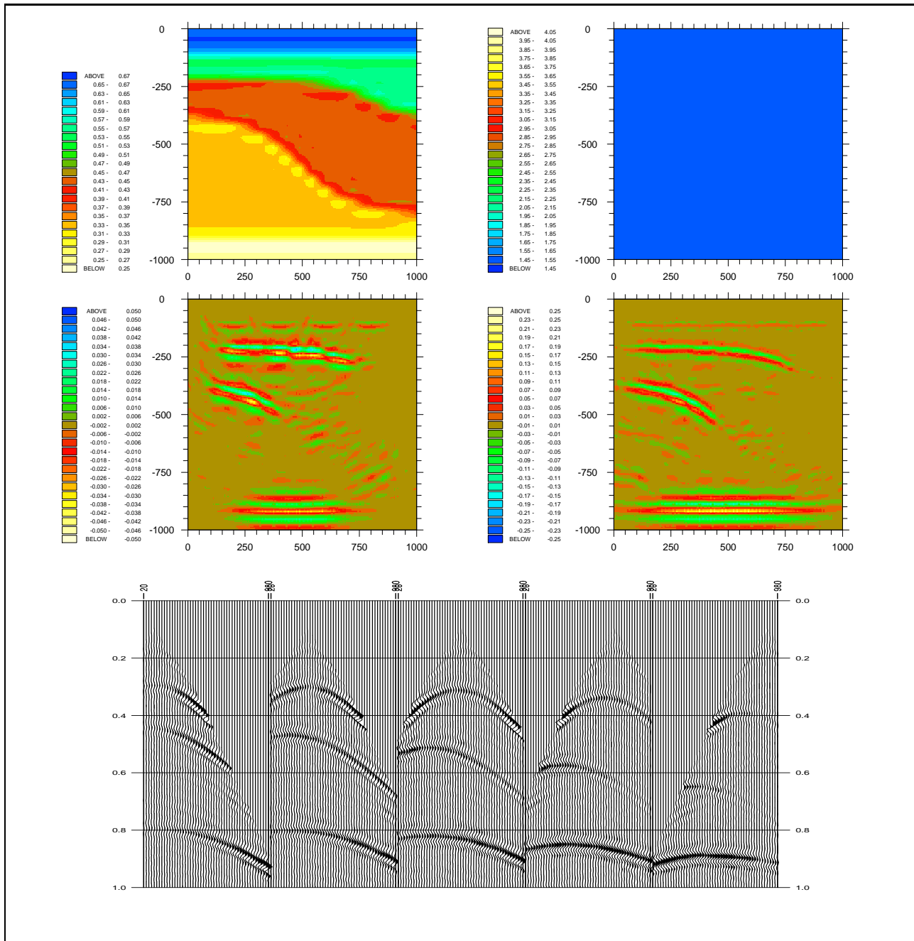
FIG. 17 – Resimulation des données pour la “vraie” lenteur lisse. Pour les sections en temps, axe horizontal : position des récepteurs, axe vertical : temps (s). Pour les sections en profondeur, axe horizontal : distance horizontale (m), axe vertical : altitude (m). Les lenteurs sont en 10^{-3} s/m et les impédances en 10^6 kg/m 2 s. Haut : “vraie” lenteur lisse \bar{v}_s (gauche) et impédance lisse constante 1,5 (droite). Milieu : estimations intermédiaires de la lenteur rugueuse r_\nu (gauche) et de l’impédance rugueuse r_\sigma (droite). Bas : simulation dans le milieu (\bar{v}_s + r_\nu; 1,5 + r_\sigma) .
