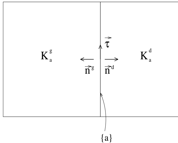
FIG. 12 – Rectangles communs à l'arête a
