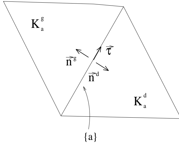
FIG. 3 – Triangles communs à l'arête a
