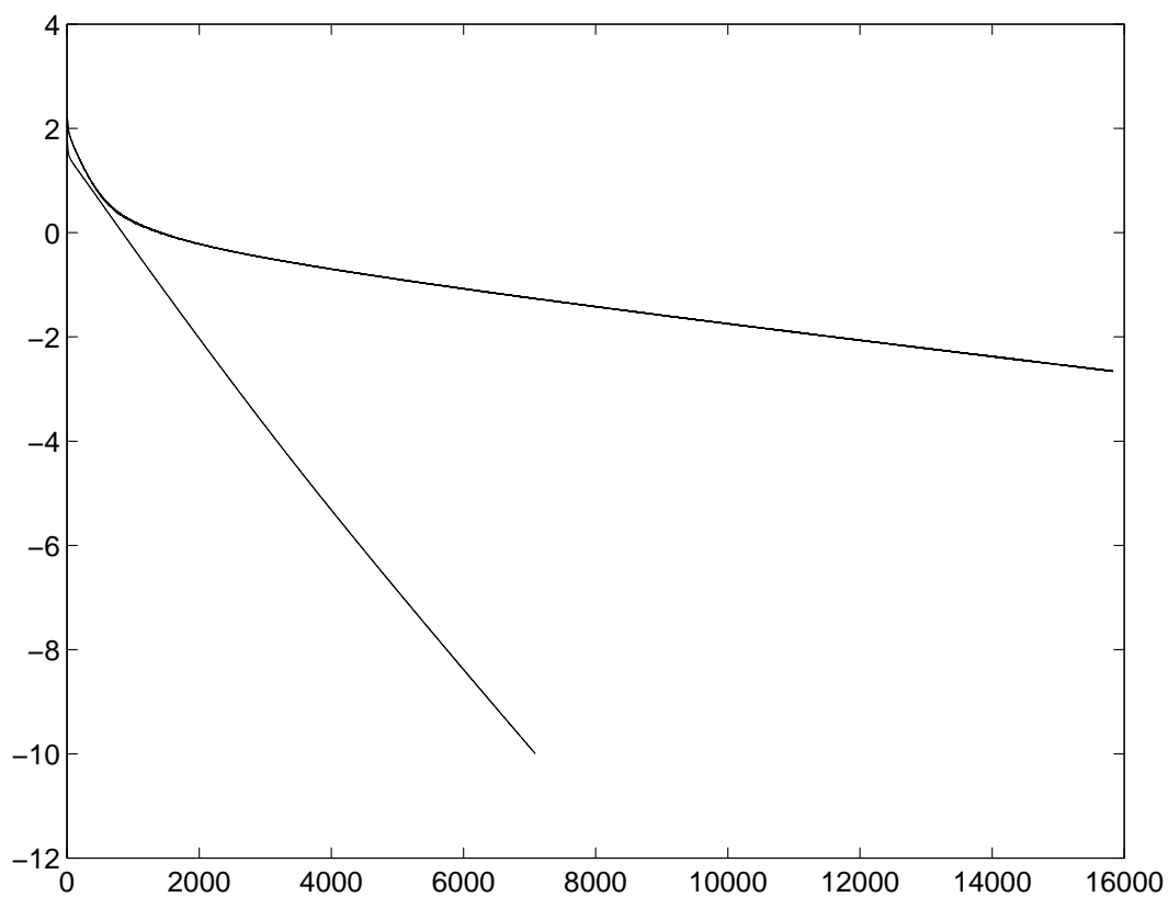
FIG. 1 - \log_{10}(\text{err}^n) en fonction de n . de haut en bas : rel = 1, 0.5 .
