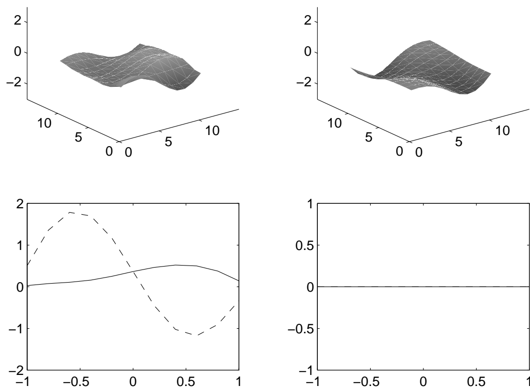
FIG. 12 – Solution au temps t = 2 s. A gauche : en haut solution contrôlée, en bas le contrôle sur les bords N et S (représentés par deux courbes. A droite : en haut solution non contrôlée, en bas pas de contrôle (0 sur les bords).
