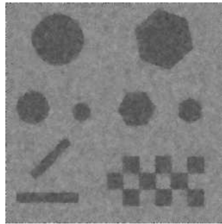
Posterior mean image
