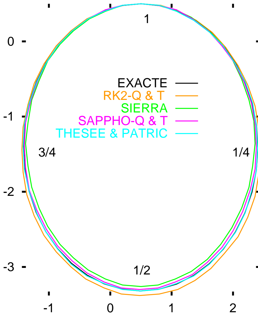
FIG.F: Parcours de la cloche dans le plan (x, y) . Instant photos. Les effets dispersifs perceptibles.
