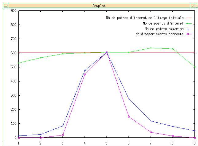
FIG. 12: Résultats de l'appariement sur la séquence du magazine, en utilisant les invariants à la seule rotation.
