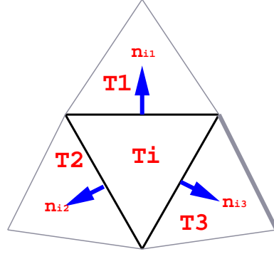
FIG. 3 – les trois voisins par arête du triangle T_i
