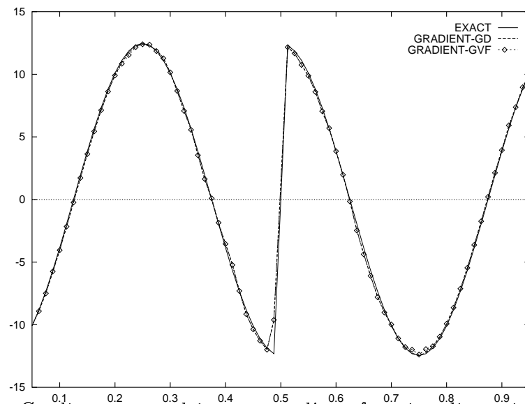
FIG. 8 – Gradients approchés et exact d'une fonction discontinue
