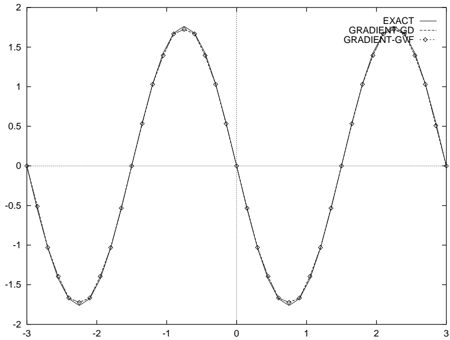
FIG. 5 – Gradients approchés et exact d'une fonction régulière
