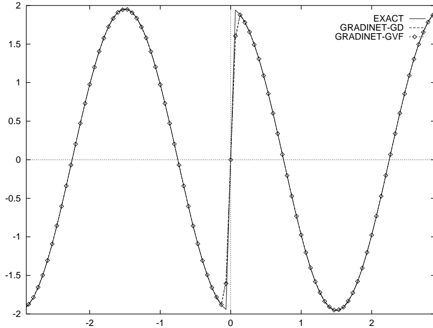
FIG. 6 – Gradients approchés et exact d'une fonction discontinue
