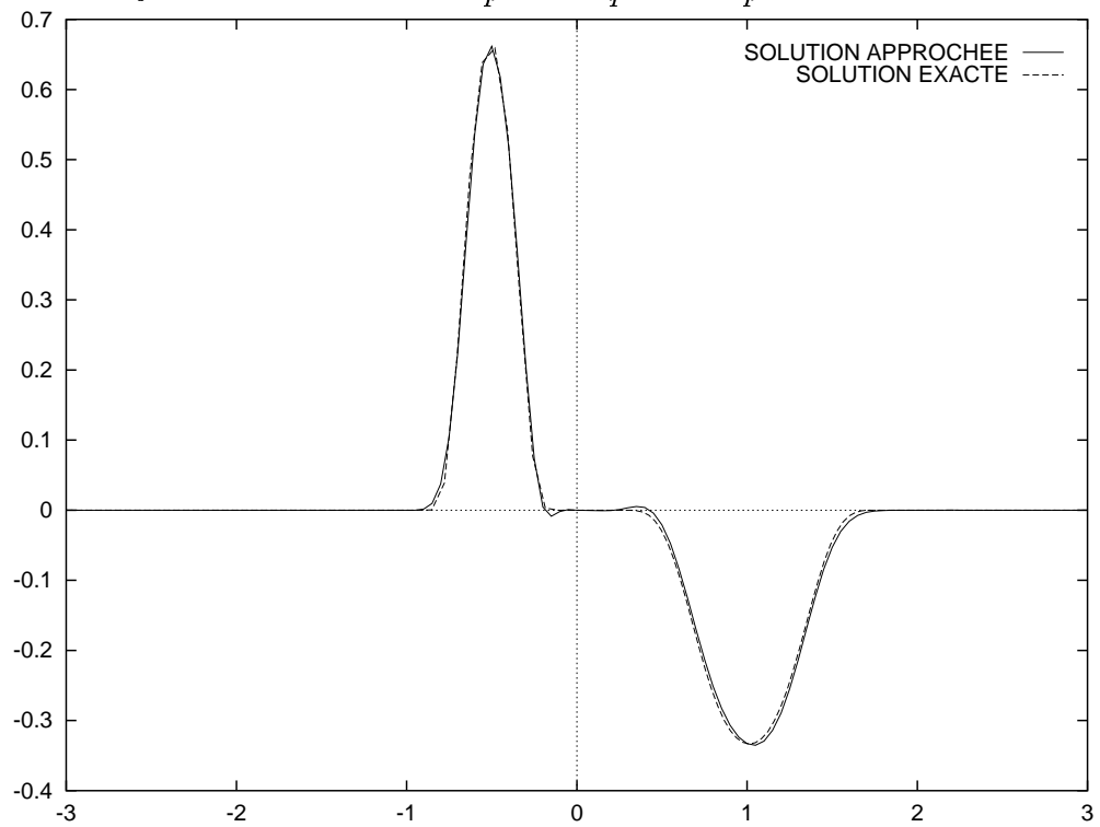
FIG. 11 – coupe en y du champ électrique après un temps t = 6.66ns
