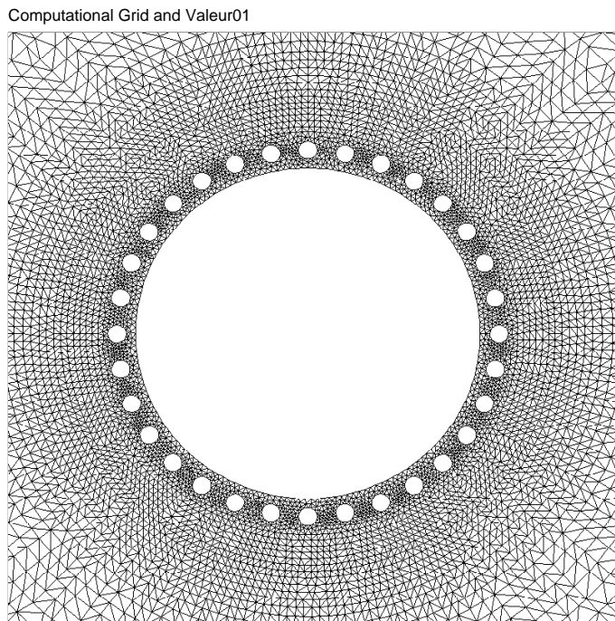
FIG. 12 – un zoom du maillage du disque revêtu
