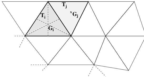
FIG. 2 – Volumes de contrôle.
