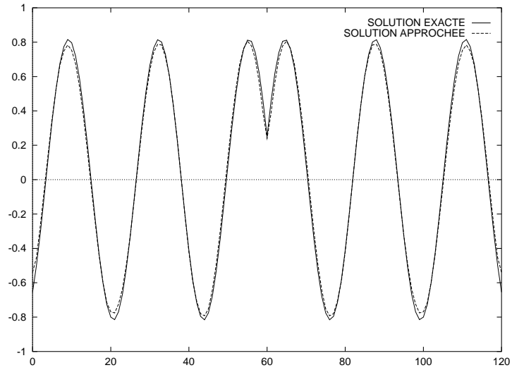
FIG. 17 – coupe en y du champ électrique
