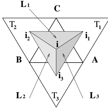
FIG. 4 – Trois candidats pour une interpolation linéaire sur (BAC) .
