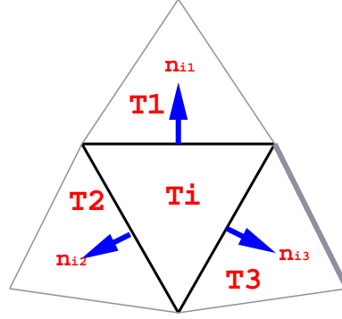
FIG. 3 – les trois voisins par arête du triangle T_i
