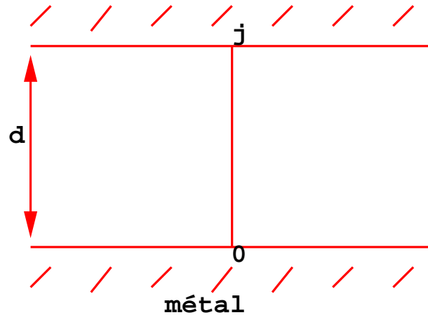
FIG. 15 – Courant surfacique dans un guide d'onde rectangulaire
