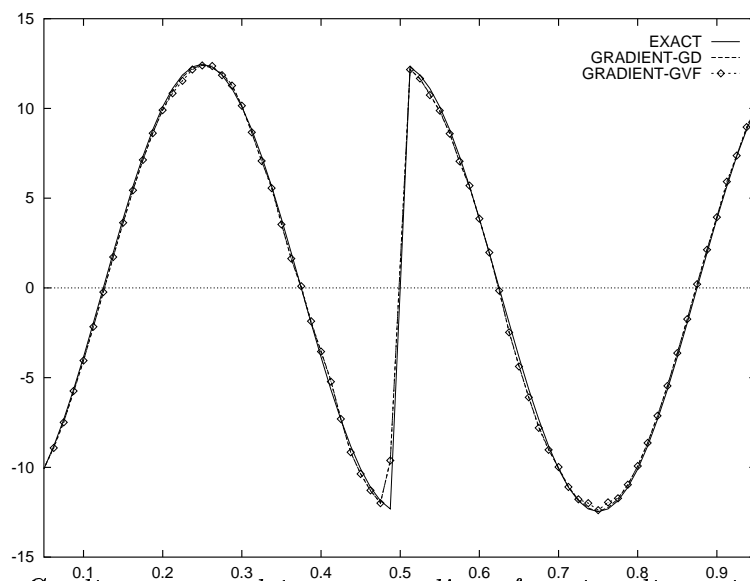
FIG. 8 – Gradients approchés et exact d'une fonction discontinue
