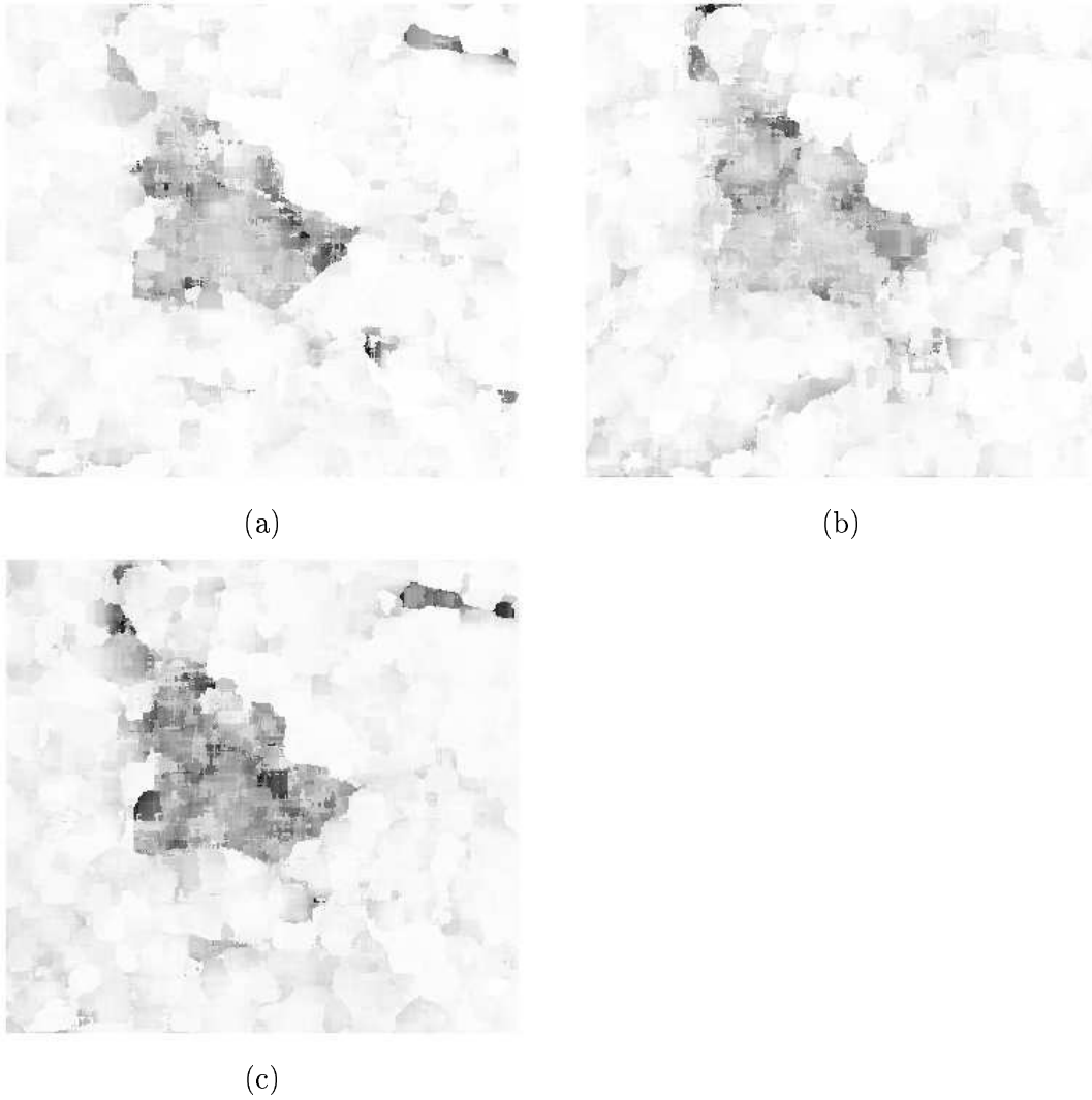
FIG. 2 – Images de l'estimée du paramètre de texture considéré (Mode vidéo inversé): (a) direction N, (b) NO et (c) modèle 2D isotrope
