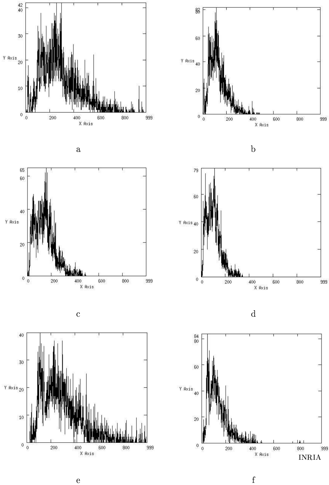
FIG. 10 – histogrammes des variances conditionnelles dans les directions (a)(b): NOn, (c)(d): NO, (e)(f): NOo ((a)(c)(e): sans correction colonne de gauche, (b)(d)(f): avec correction colonne de droite)
