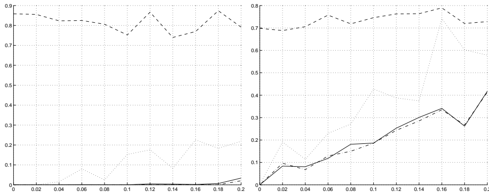
FIG. 3.4 – Erreurs en rotation (gauche) et en translation (droite) pour l'étalonnage en fonction du niveau de bruit dans le cas de 2 mouvements de faible amplitude du robot selon les différentes méthodes : axe/angle (—), quaternions (···), non-linéaire (- -), linéaire (- ·).
