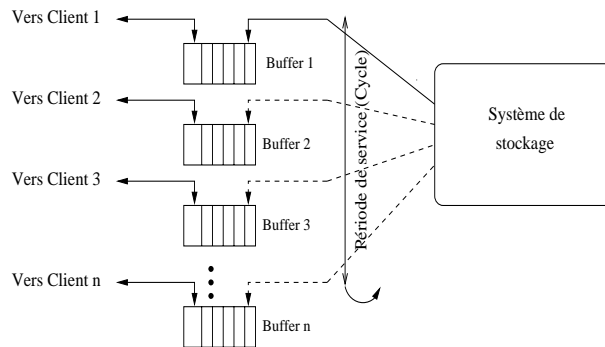
FIG. 4: Fonctionnement en cycle d'un serveur vidéo. Durant un cycle, le serveur charge, pour chaque flux, des données depuis le système de stockage vers la mémoire allouée à cet effet. Les données chargées sont ensuite consommées par les clients
