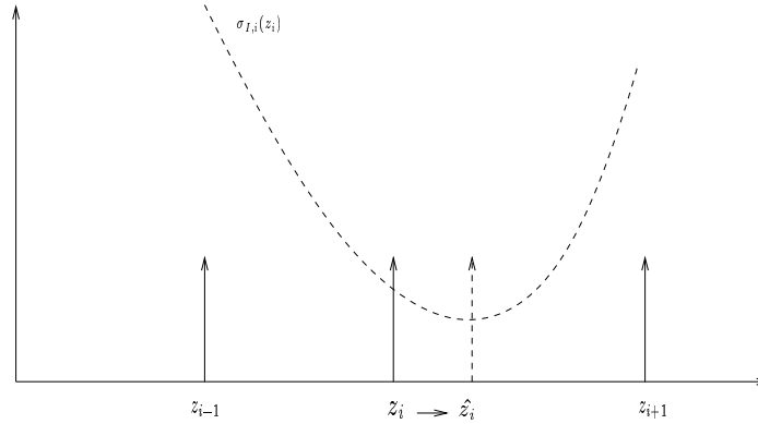
FIG. 3 – Illustration de l’algorithme d’ajustement des bornes : pour z_{i-1} et z_{i+1} fixés, la valeur optimale \hat{z}_i de z_i est celle minimisant la fonction \sigma_I(z_i)
