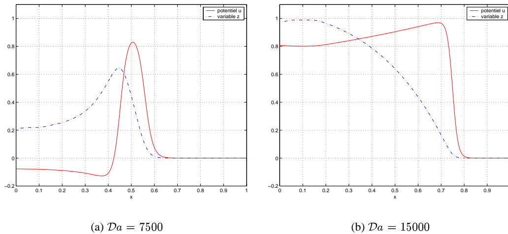
FIG. 1.14 – Comportement des solutions pour différentes valeurs de Da
