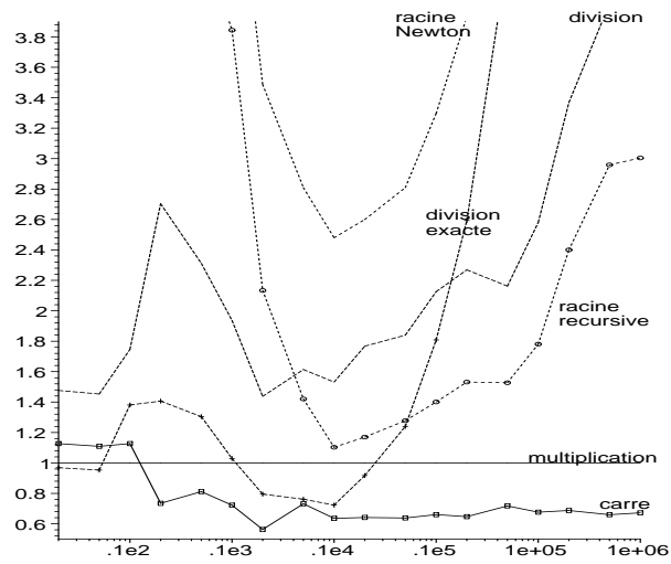
FIG. 2. Comparaison de différentes opérations sur les entiers en GMP 3.1.1 sur un Pentium II. L'abscisse indique le nombre n de chiffres décimaux des opérands, l'ordonnée le rapport des temps par rapport à la multiplication n \times n
