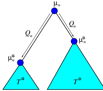
FIG. 7: Modèle d'évolution sur un arbre enraciné T : une loi \mu est associée à la racine r(T) , un générateur infinitésimal Q est associé à la descendance gauche ainsi qu'à la droite (le même générateur pour les deux). Indépendamment, on associe alors une loi \mu^G (resp. \mu^D ) à la racine T^G (resp. T^D ). La propagation de la loi initiale \mu se fait indépendamment le long des branches de T .
